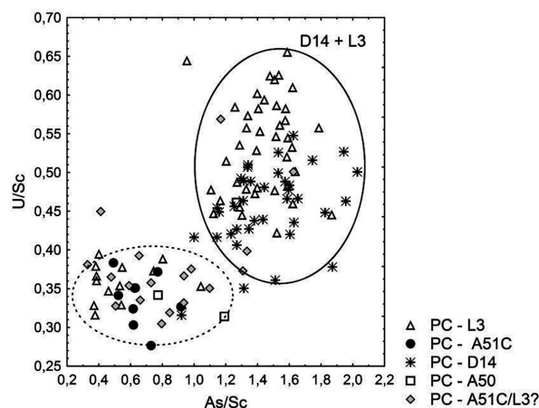
Fig. 8 – As/Sc vs U/Sc segundo as tipologias das ânforas do centro produtor de PC, evidenciando duas grandes tendências composicionais.
