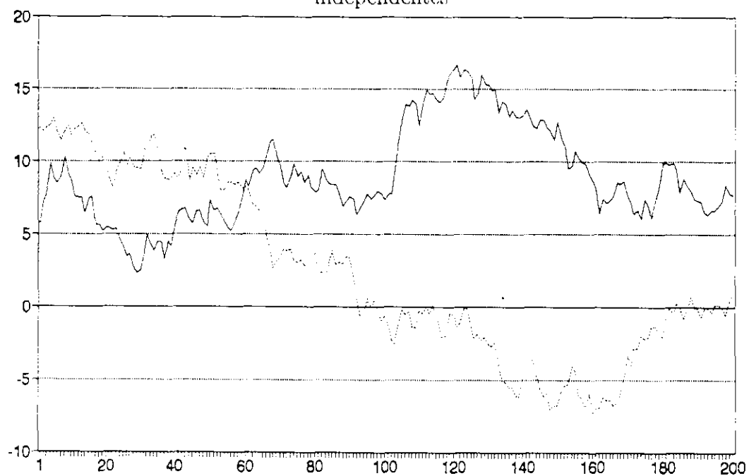
Gráfico 4 Inexistência de cointegração entre séries I(1) : passeios aleatórios independentes
