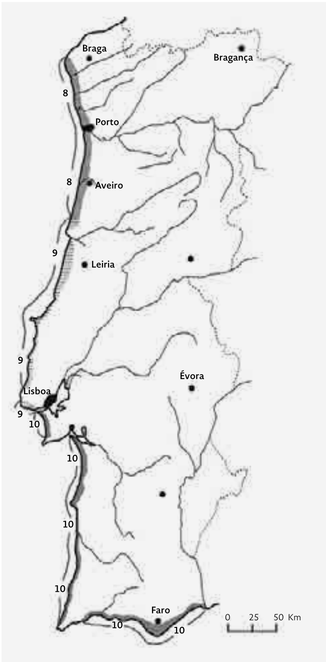
FIGURA 8 Duna cinzenta (duna penestabilizada) – Vegetação arbustiva baixa (camefítica). Associações e habitats da Rede Natura. Associações Habitats 8 Iberidetum procumbentis 2130* 9 Armerio welwitschii - Crucianelletum maritimae 2130* 10 Artemisio crithmifoliae - Armerietum pungentis 2130*
