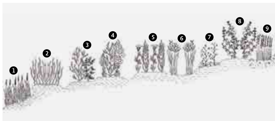
FIGURA 6 Geopemasigmetum do rio Mira junto à ponte de Vila Nova de Milfontes (Odemira): 1 Spartinetum maritimae ; 2 Puccinellio ibericae - Sarcocornietum perennis ; 3 Halimione portulacoidis - Sarcocornietum alpinum ; 4 Cistancho phelypaeae - Sarcocornietum pruinosae ; 5 Inulo crithmoidis - Arthrocnemum macrostachyi ; 6 Polygono equisetiformis - Juncetum maritimi ; 7 Limonietum lanceolati ; 8 Cistancho phelypaeae - Suaedetum verae ; 9 Comunidade de Spartina patens . [Extraído e modificado a partir de Neto, Arsénio & Costa (2009b).]
