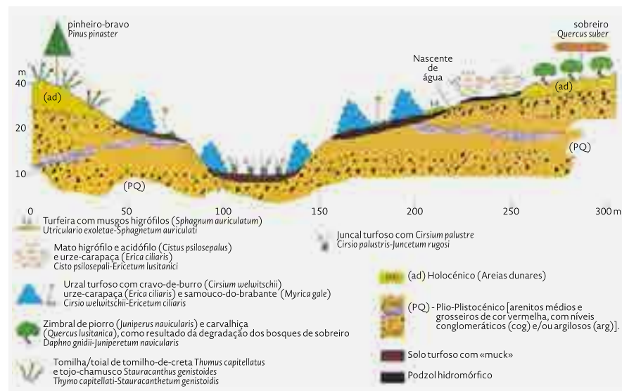
FIGURA 9 Transecto realizado num complexo turfoso no Moinho da Ordem (Alcácer do Sal). A água é proveniente do aquífero que se forma na base das dunas (paleodunas), no contacto com a superfície plioptocénica constituída por arenitos, conglomerados e níveis argilosos. No complexo psamófilo do lado esquerdo, em dunas de grande profundidade a maior aridez leva ao desenvolvimento de comunidades da Saturacantho-Halimietalia , enquanto, do lado direito, a menor espessura das dunas permite uma maior proximidade da toalha freática da superfície e a ocorrência dos sobreirais sobre areias ( Aro neglecti-Quercetum suberis ) e a original associação ( Daphne-Juniperetum naucularis ). O complexo palustre e turfoso é formado por um conjunto de comunidades de grande originalidade, a maioria das quais relictas, cuja proteção e conservação é urgente, dada a velocidade de extinção destes habitats , principalmente devido a mudanças de ocupação e uso do solo. [Extraído e modificado a partir de Moreira & Neto, 2005.]
