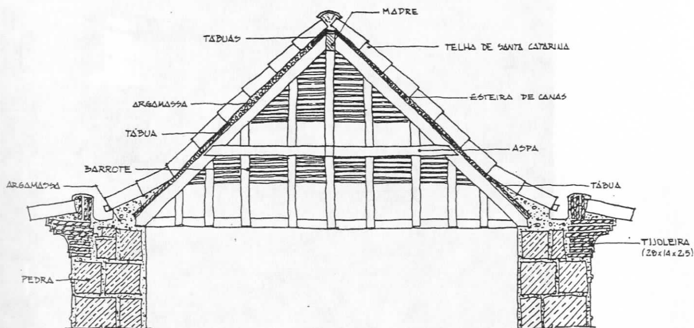
CORTE ESQUEMÁTICO DE TELHADO DE TESOURO
