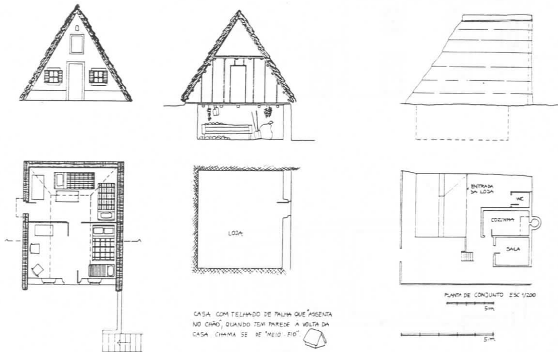
FIG.300 - Ilha da Madeira, casa em Santana. Levantamento do autor, 1986 Esc. 1/200
