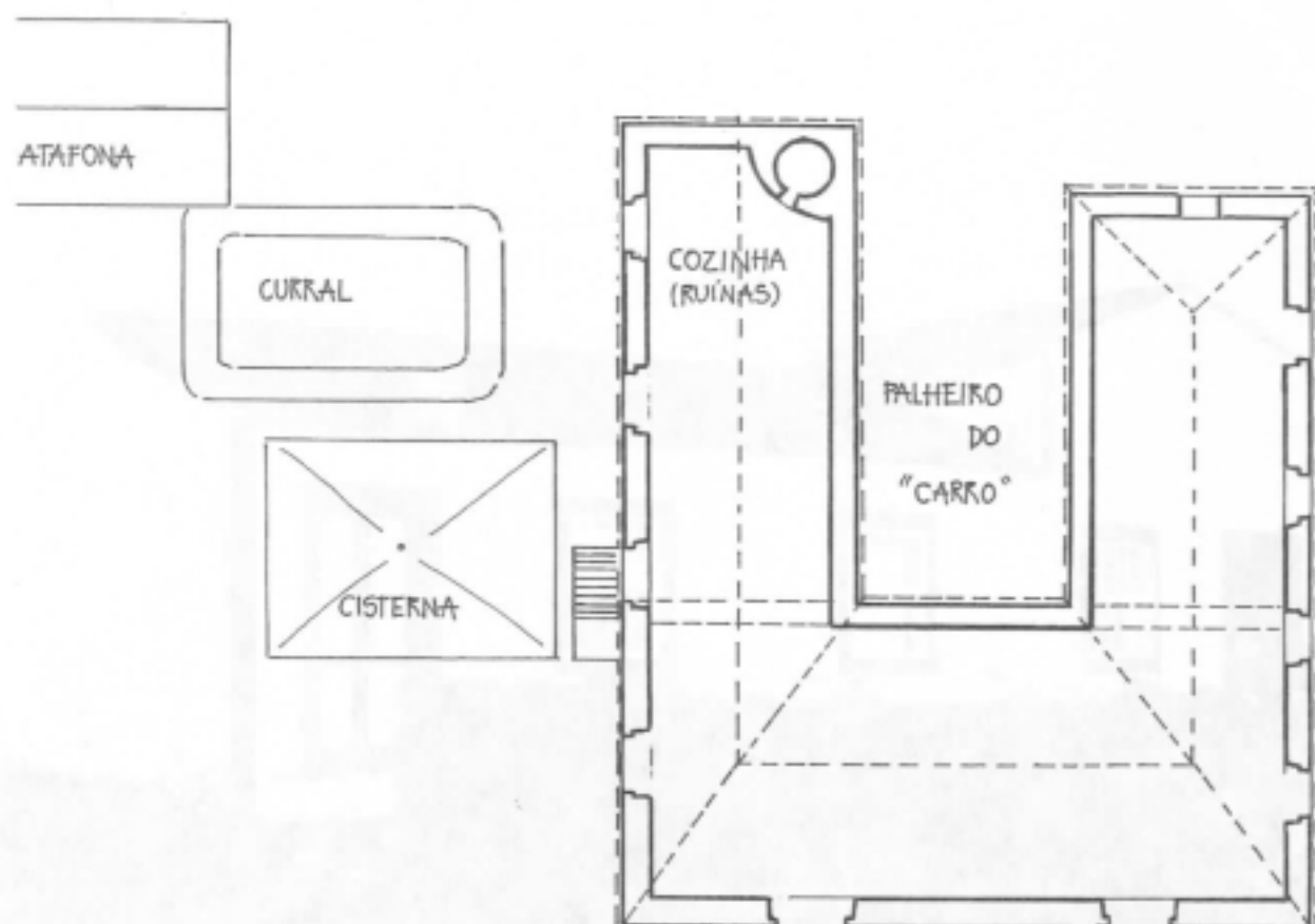
FIG.294 - Ilha do Pico, São Roque: solar com a disposição da planta em "U". In FERNANDES [et. al.] [210] Açores, s/ n. ficha. Levantamento
