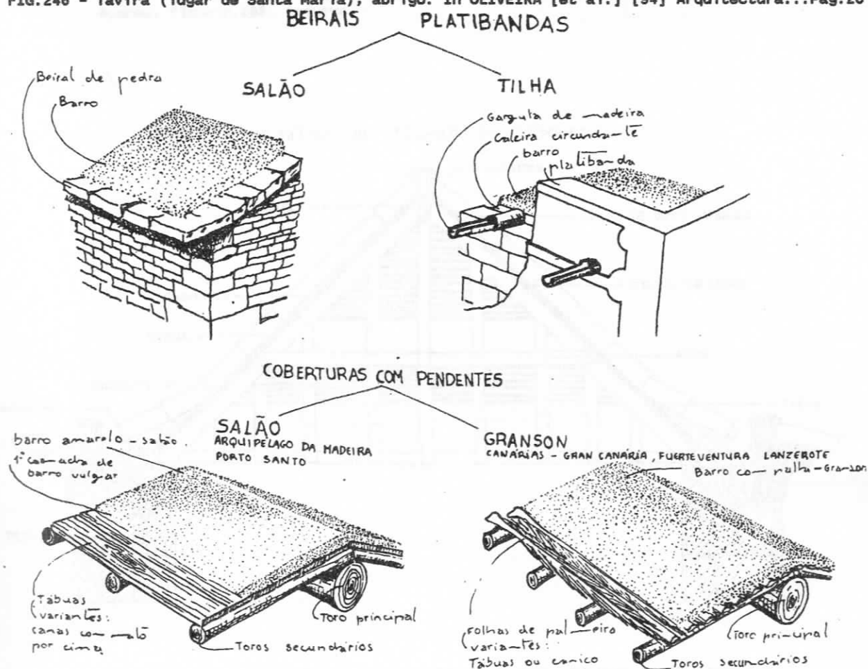
FIG.247 - Porto Santo e Canárias: coberturas de tipo "salão" e "granson". In MESTRE [181], Pág.5
