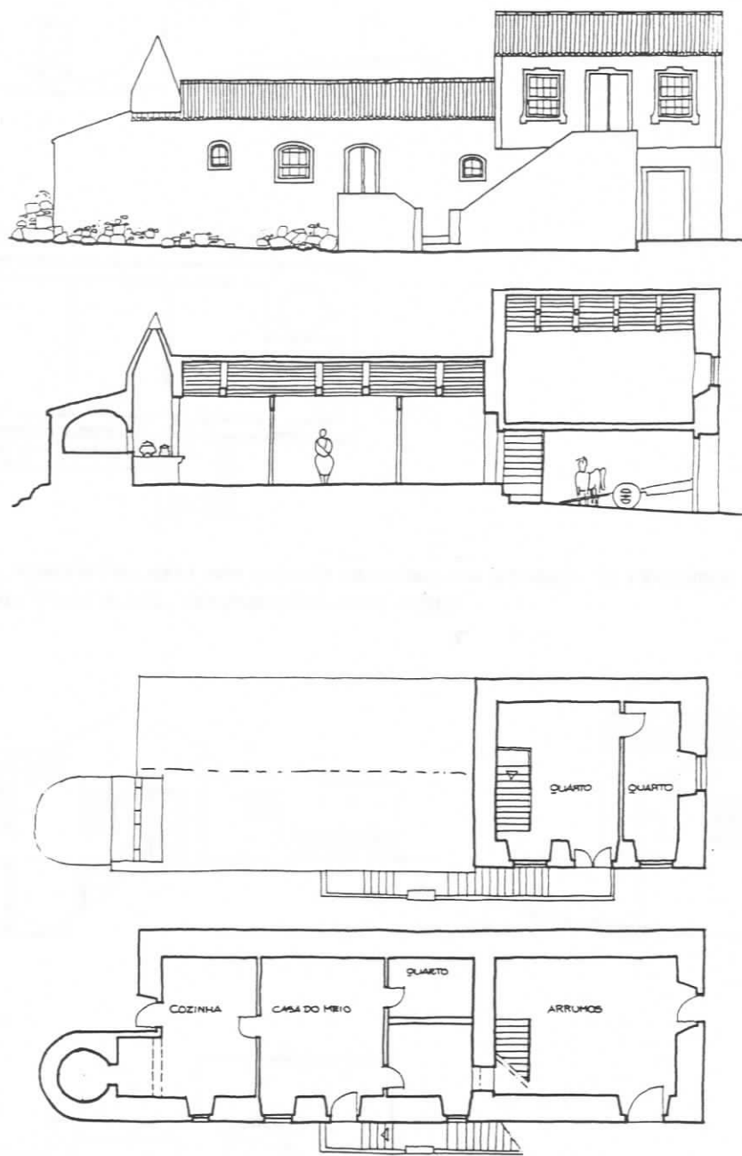
FIG.327 - Terceira, Feteira. In FERNANDES [et al.] [210] Açores, ficha n.29. Arquivo. Esc. 1/200
