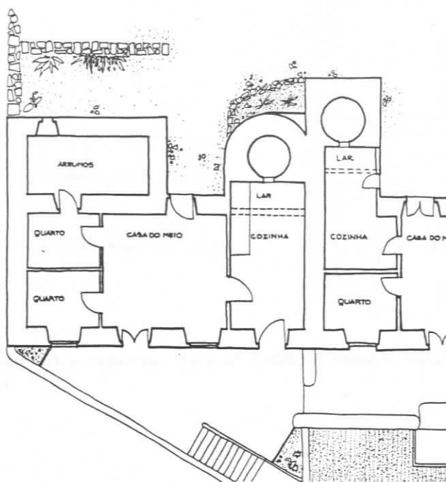
FIG.342 - Terceira, São Sebastião. In FERNANDES [et al.] [210] Açores, ficha n.40, Arquivo. Esc. 1/200
