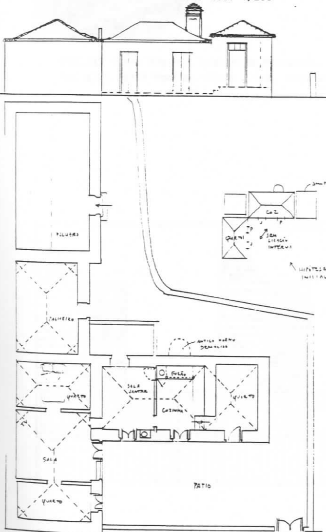
FIG.315 - La Palma, El Paso. In FERNANDES [213] Canárias, ficha n.312 Esc. 1/200
