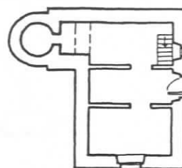
FIG.339 - São Miguel, Mosteiros. In FERNANDES [et al.] [210] Açores, ficha n.32. Arq.Esc.1/200
