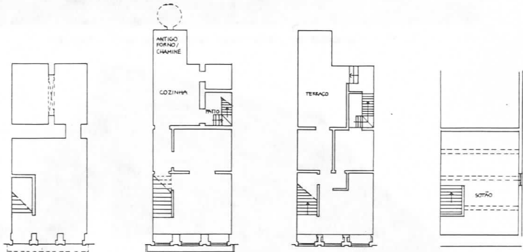
FIG.238 - Angra, casa na rua do Galo. In FERNANDES [153] Angra...pág.76 Esc. 1/200
