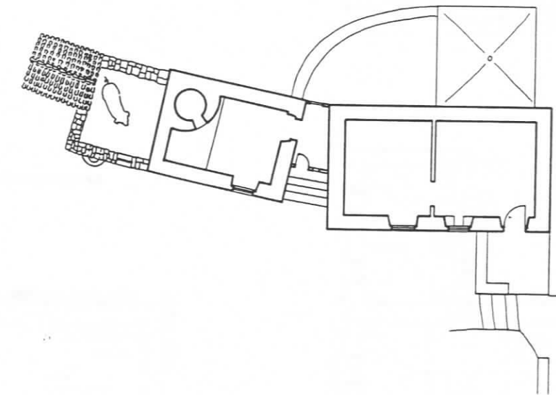
FIG.304 - Ilha do Pico, Terra do Pão. In FERNANDES [et al.] [210] Açores, ficha n. 111. Levantamento. Esc. 1/200
