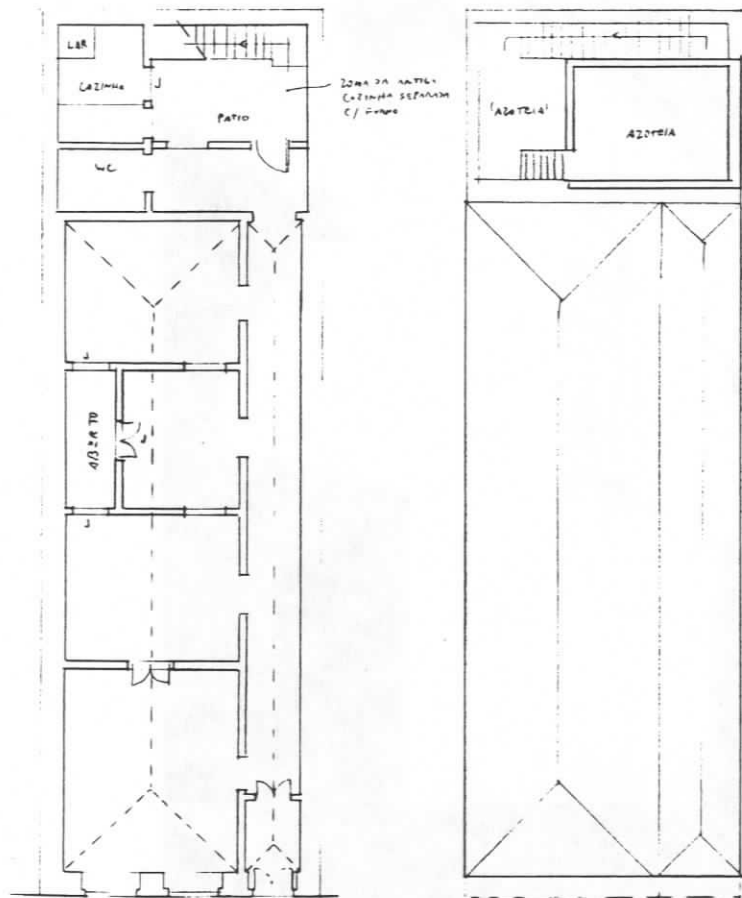
FIG.219 - La Palma, Santa Cruz. In FERNANDES [213] Canárias, ficha n.50 Esc. 1/200
