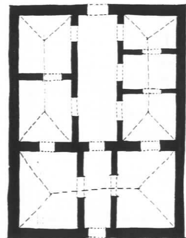
FIG.316 - Cabo Verde, ilha de Maio, Barreiro. In POURBAIX [186] Culture... pág.100 Esc. 1/200
