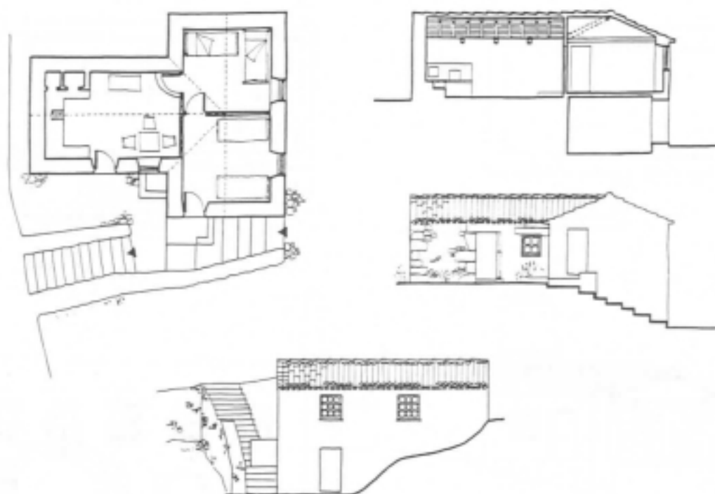
FIG.319 - São Jorge, Norte Grande: casa com planta "em T". In FERNANDES [et al.] [210] Açores, ficha n.38. Esc. 1/200
