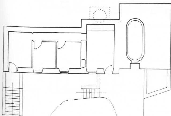
FIG.331 - Pico, Calheta do Nesquim. In FERNANDES [et al.] [210] Açores, ficha n.87. Levantamento. Esc. 1/200
