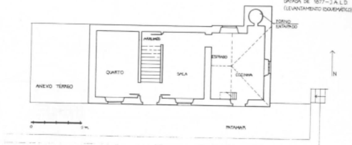
FIG.334 - Porto Santo, Vila Baleira. In FERNANDES, José Manuel; JANEIRO, Maria de Lurdes [163] Arquitectura... pág.53. esc. 1/200
