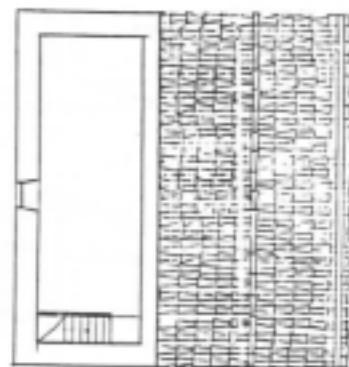
FIG.348 - São Miguel, Feteira Pequena, Santana. In FERNANDES [et al.] [210] Açores, ficha n.524. Levantamento. Esc. 1/200
