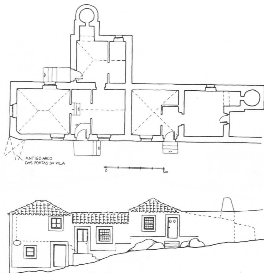
FIG.223 - Santa Maria, Vila do Porto. In FERNANDES [et al.] [210] Açores, ficha n.30 Arquivo Esc. 1/200
