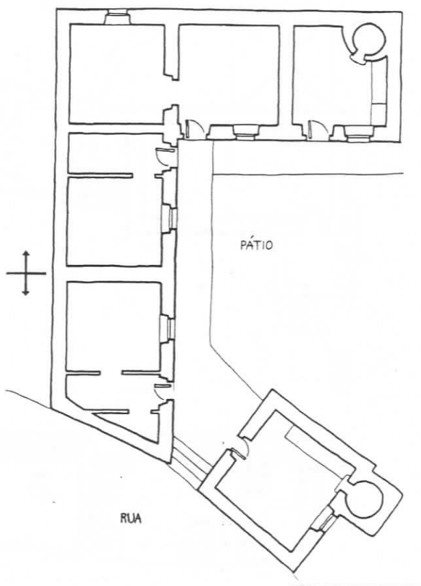
FIG.303 - São Miguel, Nordeste. In FERNANDES [et al.] [210] Açores, ficha n.515 A. Levantamento. Esc. 1/200
