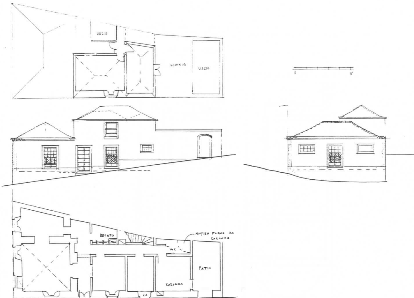
FIG.225 - La Palma, Santa Cruz. In FERNANDES [213] Canárias, ficha n.253 Esc. 1/200
