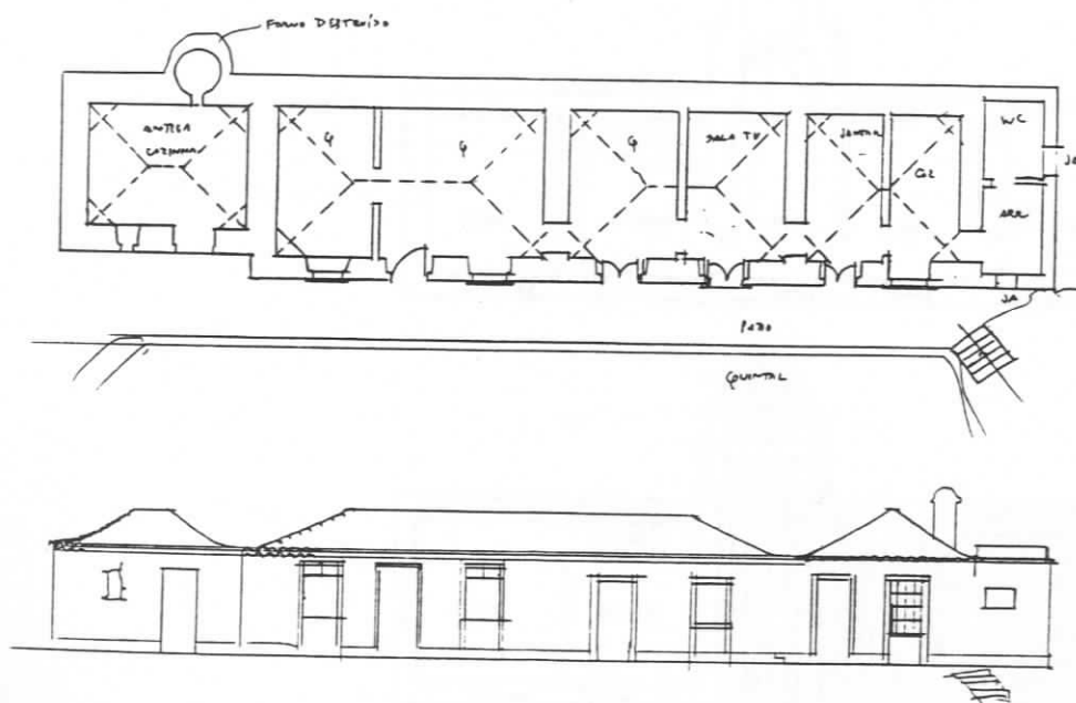
FIG.333 - La Palma, Puntallana. In FERNANDES [213] Canárias, ficha n.280. Esc. 1/200
