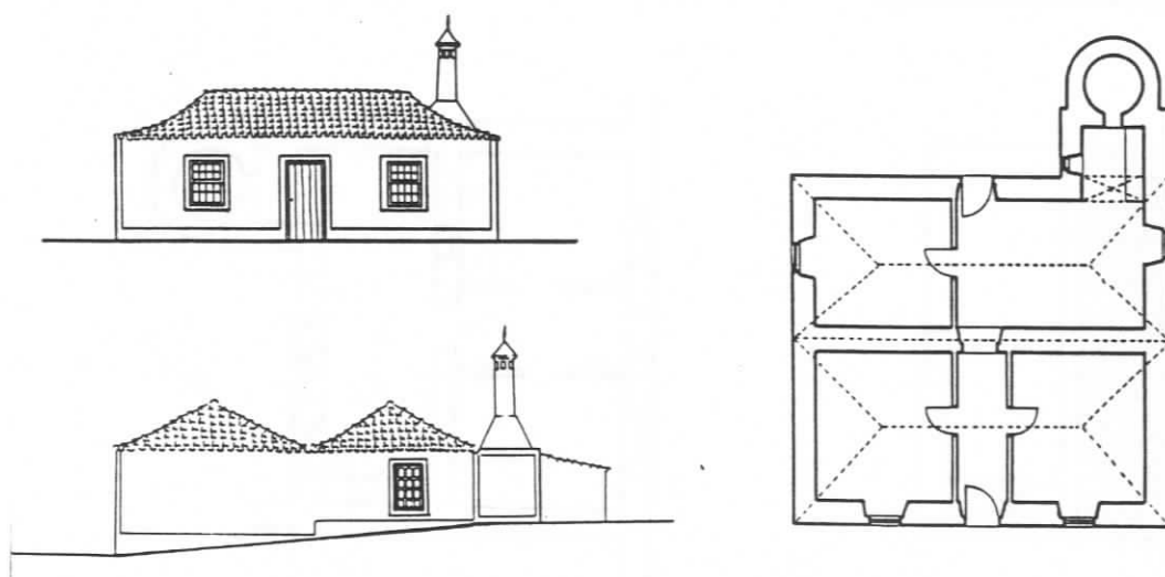
FIG.346 - Santa Maria, Chã de São Tomé. In FERNANDES [et al.] [210] Açores, ficha n.47. Arquivo. Esc. 1/200
