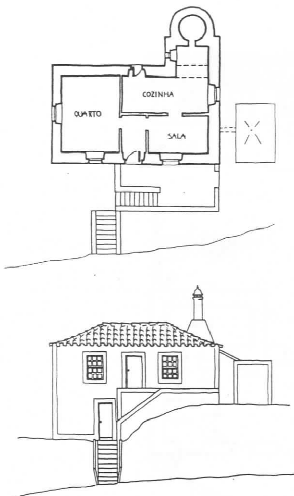
FIG.338 - Santa Maria, Arrebetão In FERNANDES [et al.] [210] Açores, ficha n.69. Arquivo. Esc.1/200
