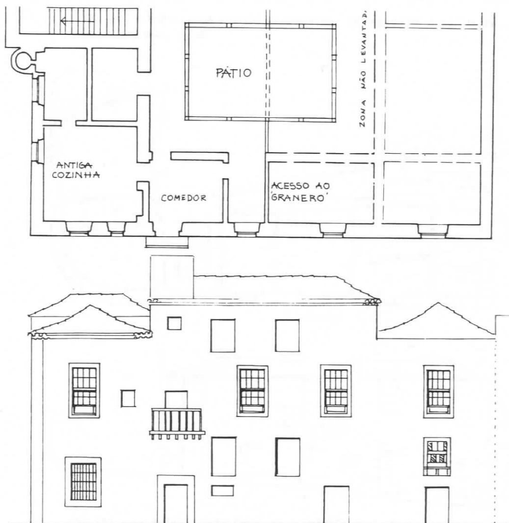
FIG.229 - La Palma, Santa Cruz. In FERNANDES [66] O Lugar... pág.102 Esc. 1/200
