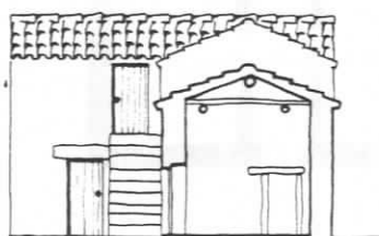
FIG.313 - Corvo, Vila Nova do Corvo. In FERNANDES [et al.] [210] Açores, ficha n.3. Arquivo. Esc. 1/200
