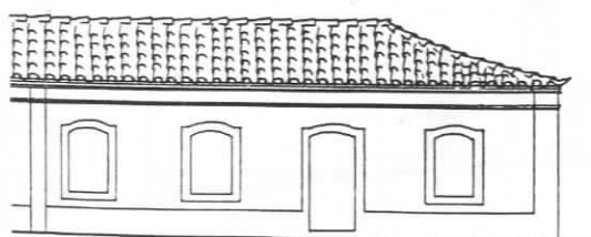
FIG. 344 - Algarve, arr. de Monchique. Levantamento do autor, 1987 Esc. 1/200
