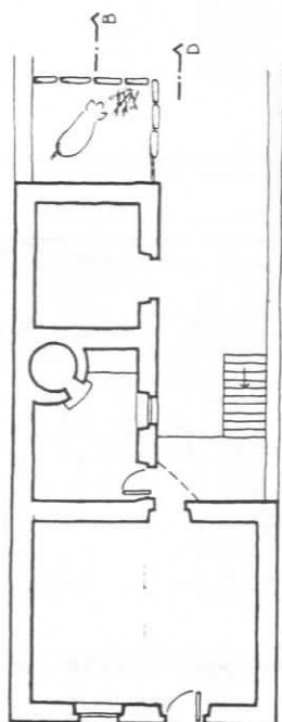
FIG.312 - São Miguel, Agua Retorta. In FERNANDES [et al.] [210] Açores, ficha n.218. Arquivo. Esc. 1/200
