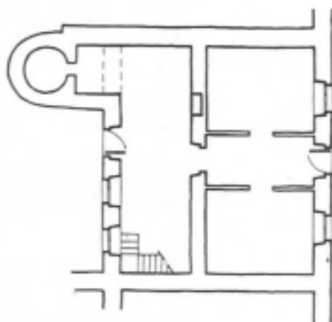
FIG.348 - São Miguel, Feteira Pequena, Santana. In FERNANDES [et al.] [210] Açores, ficha n.524. Levantamento. Esc. 1/200
