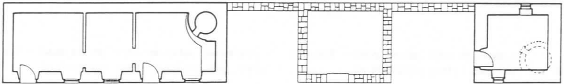
FIG.304 - Ilha do Pico, Terra do Pão. In FERNANDES [et al.] [210] Açores, ficha n. 111. Levantamento. Esc. 1/200
