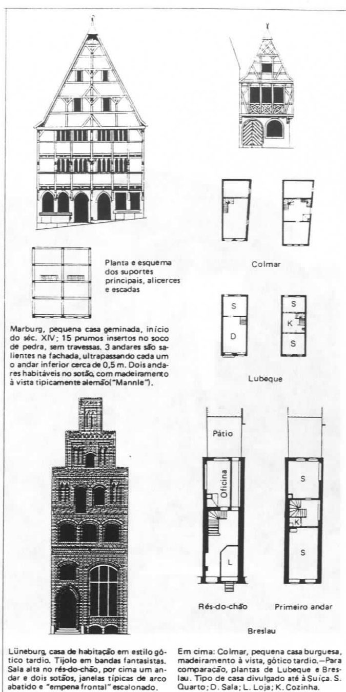
FIG.116 - Exemplificações de "arquitecturas de madeira" na Europa. In KOCH [204] Estilos...págs.95-96
