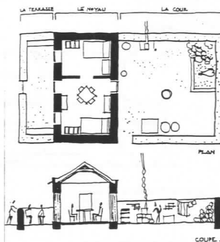
Plan et coupe du modèle rectangulaire. Source : Jeanne et Rosé & Schmitt, Habitat spontané, Praia, p.62.
