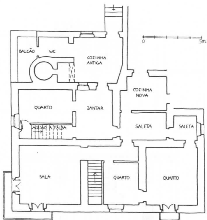
FIG.234 - São Miguel, Ribeira Grande. In FERNANDES [et al.] [210] Açores, ficha n.156 Arquivo. Esc. 1/200
