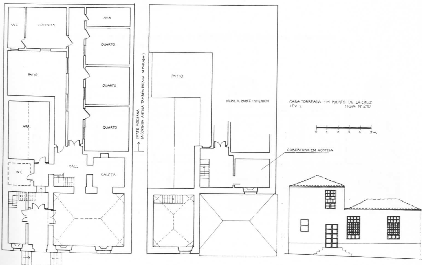
FIG.224 - Tenerife, Puerto de 1a Cruz. In FERNANDES [213] Canárias, ficha n.210. Esc. 1/200
