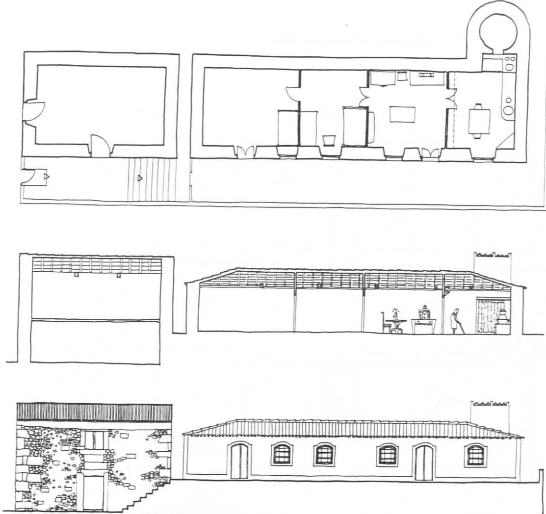
FIG.332 - Terceira, São Brás. In FERNANDES [et al.] [210] Açores, ficha n.64. Arquivo. Esc. 1/200
