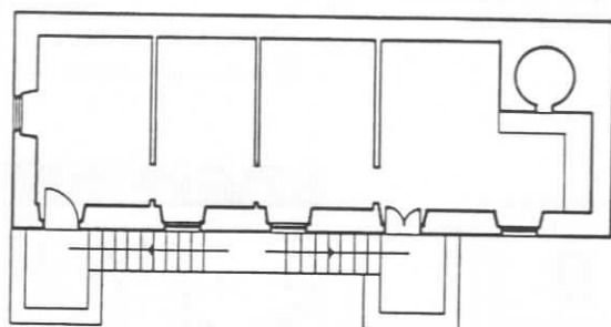
FIG.330 - Pico, Almagreira, casa com cozinha de cobertura alteada. In FERNANDES [et al.] [210] Açores, ficha n.102. Levantamento. Esc. 1/200
