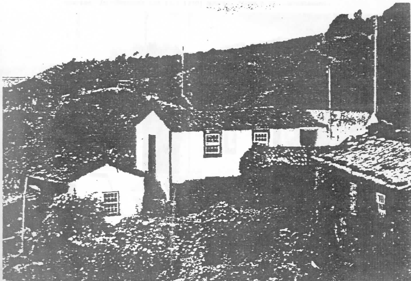
FIG.291 - Ilha do Pico, Silveira: casa com cozinha separada, tendo à direita os quartos e à esquerda a cozinha. In FERNANDES [et al.] [210] Açores, ficha n.105. Levantamento
