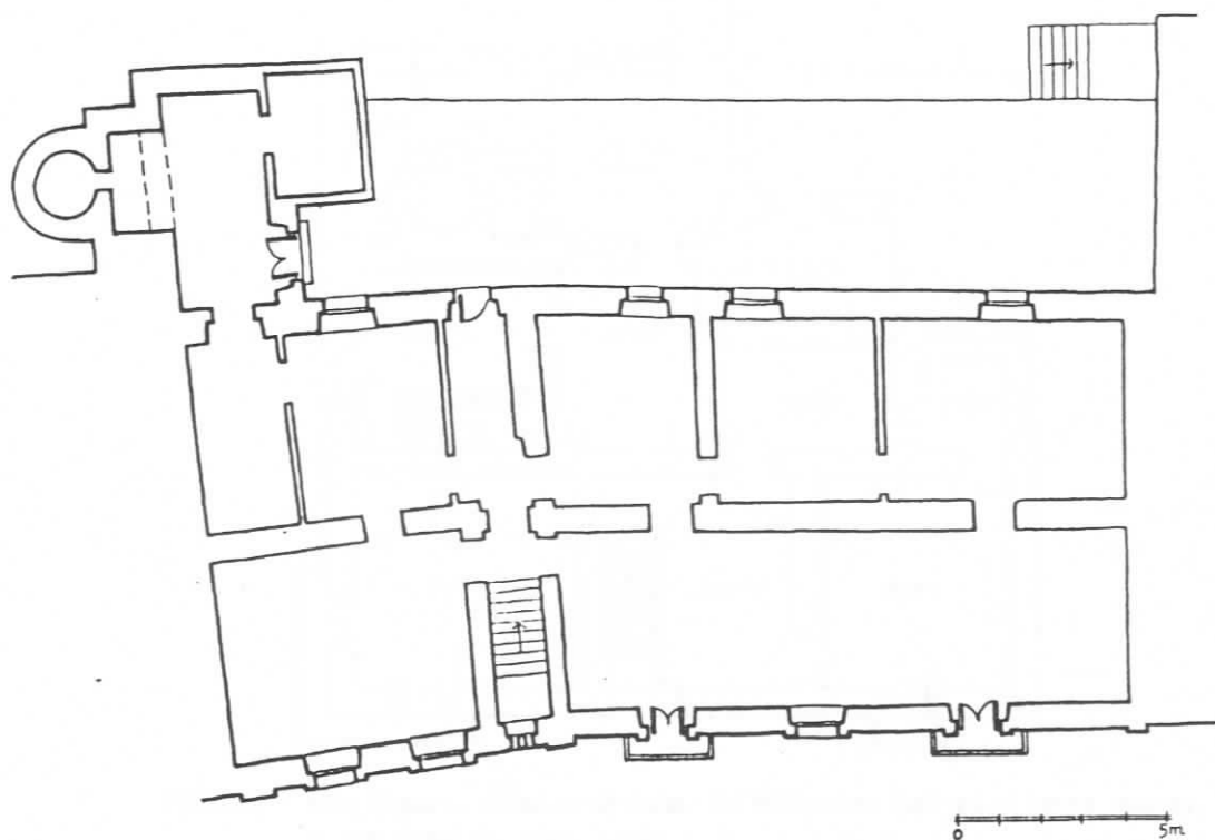
FIG.232 - São Miguel, Ribeira Grande. In FERNANDES [et al.] [210] Açores, ficha n.166 Arquivo. Esc. 1/200
