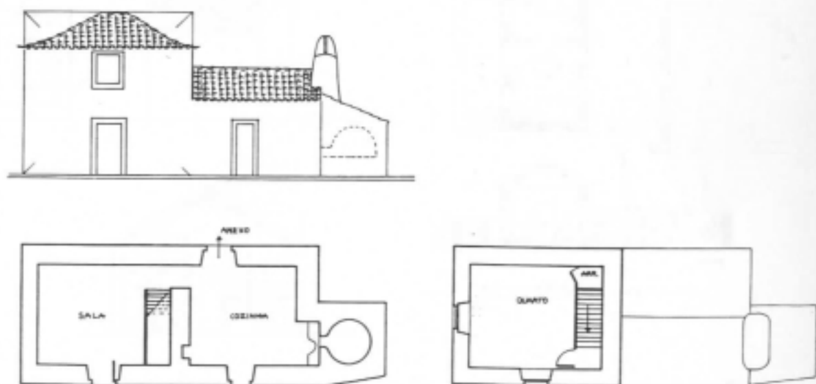
FIG.337 - Sintra, Lourel. In FERNANDES, José Manuel; JANEIRO, Maria de Lurdes [163] Arquitectura...pág.34. Esc. 1/200
