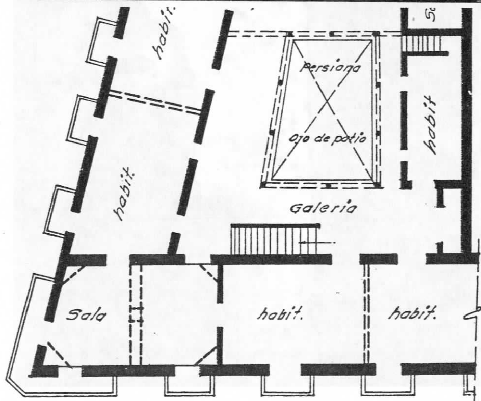
FIGS.178 e 179 - Havana, Cuba: edificio de esquina c/Obra Pia e c/ Oficios. Planta piso superior in WEISS [193] Arquitectura Cubana... pág.71. Esc. aprox. 1/200
