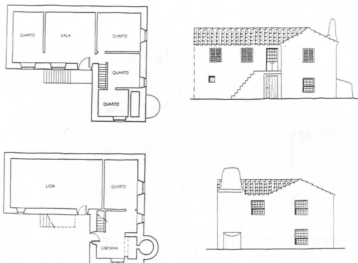
FIG.321 - Flores, Mosteiro. In FERNANDES [et al.] [210] Açores, ficha n.37. Levantamento. Esc. 1/200
