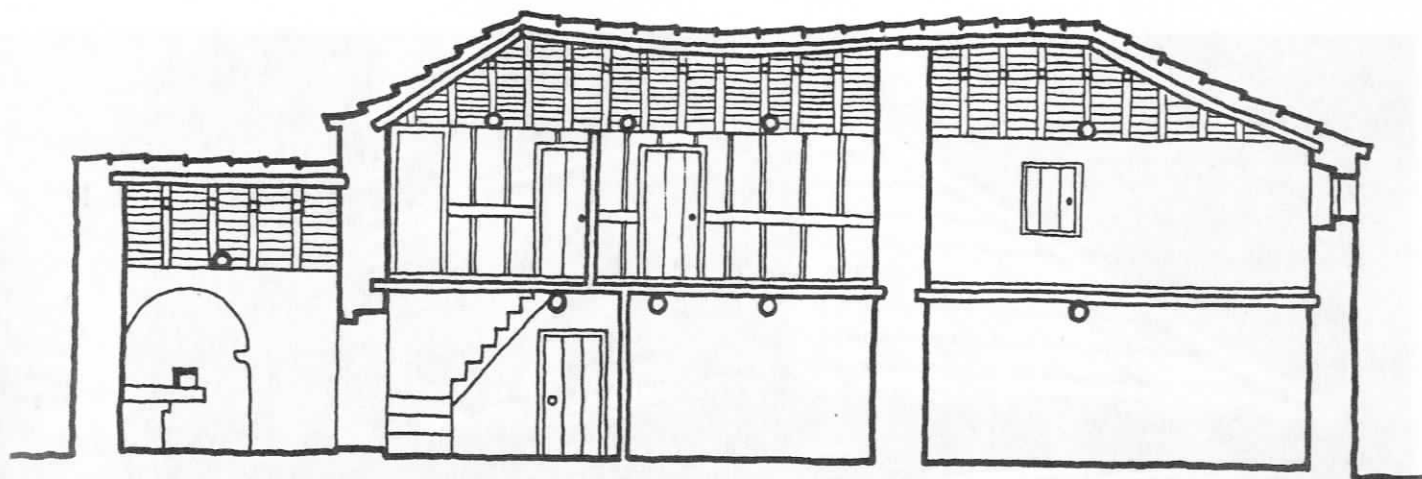
FIG. 250 - Santa Maria, Anjos. In FERNANDES [et al.] [210] Açores, ficha n.42. Arquivo. Esc. 1/100
