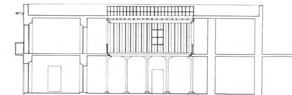
CORTE AB
