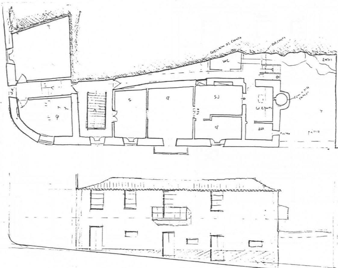
FIG.231 - La Palma, Santa Cruz. In FERNANDES [213] Canárias, ficha n.224 B1 Esc. 1/200
