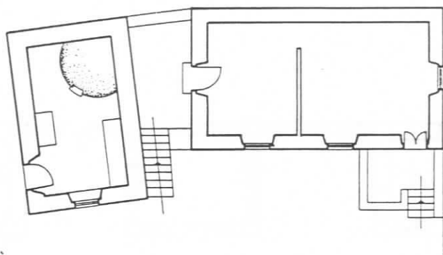
FIG.302 - Ilha do Pico, casa em Silveira. In FERNANDES [et al.] [210] Açores, ficha n.105. Levantamento Esc. 1/200
