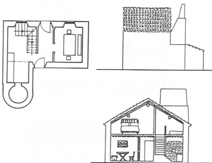
FIG.340 - São Miguel, Sete Cidades In FERNANDES [et al.] [210] Açores, ficha n.4. Arquivo. Esc.1/200
