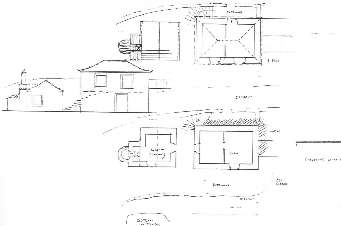
FIG.300 - Ilha da Madeira, casa em Santana. Levantamento do autor, 1986 Esc. 1/200
