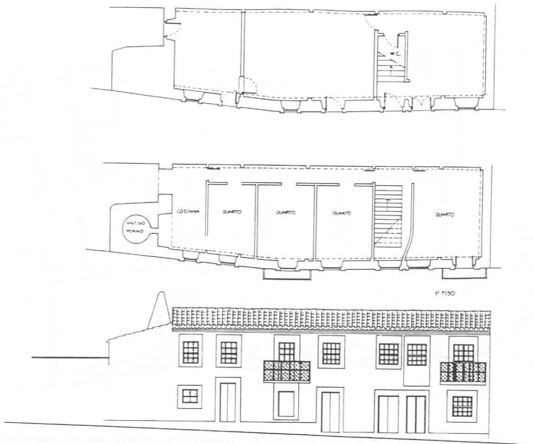
FIG. 230 - Angra, casa na rua do Cruzeiro. In FERNANDES [153] Angra...pág.74 Esc. 1/200
