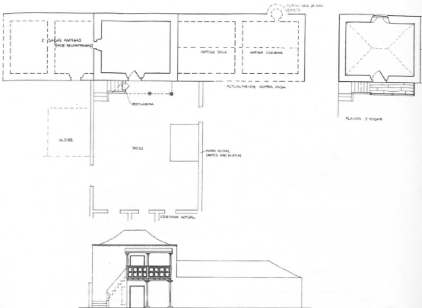
FIG.336 - Lanzarote, San Bartolomé. In FERNANDES [213] Canárias, ficha n.88. Esc. 1/200
