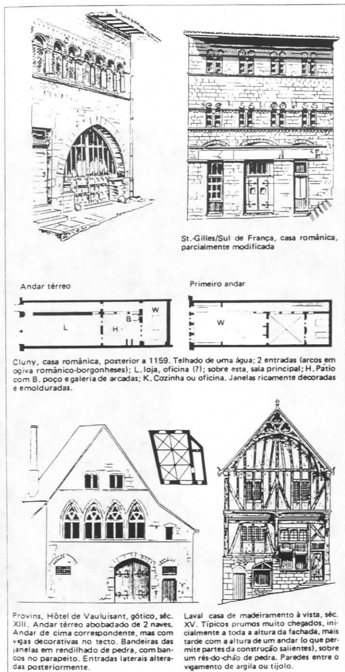
FIG.116 - Exemplificações de "arquitecturas de madeira" na Europa. In KOCH [204] Estilos...págs.95-96
