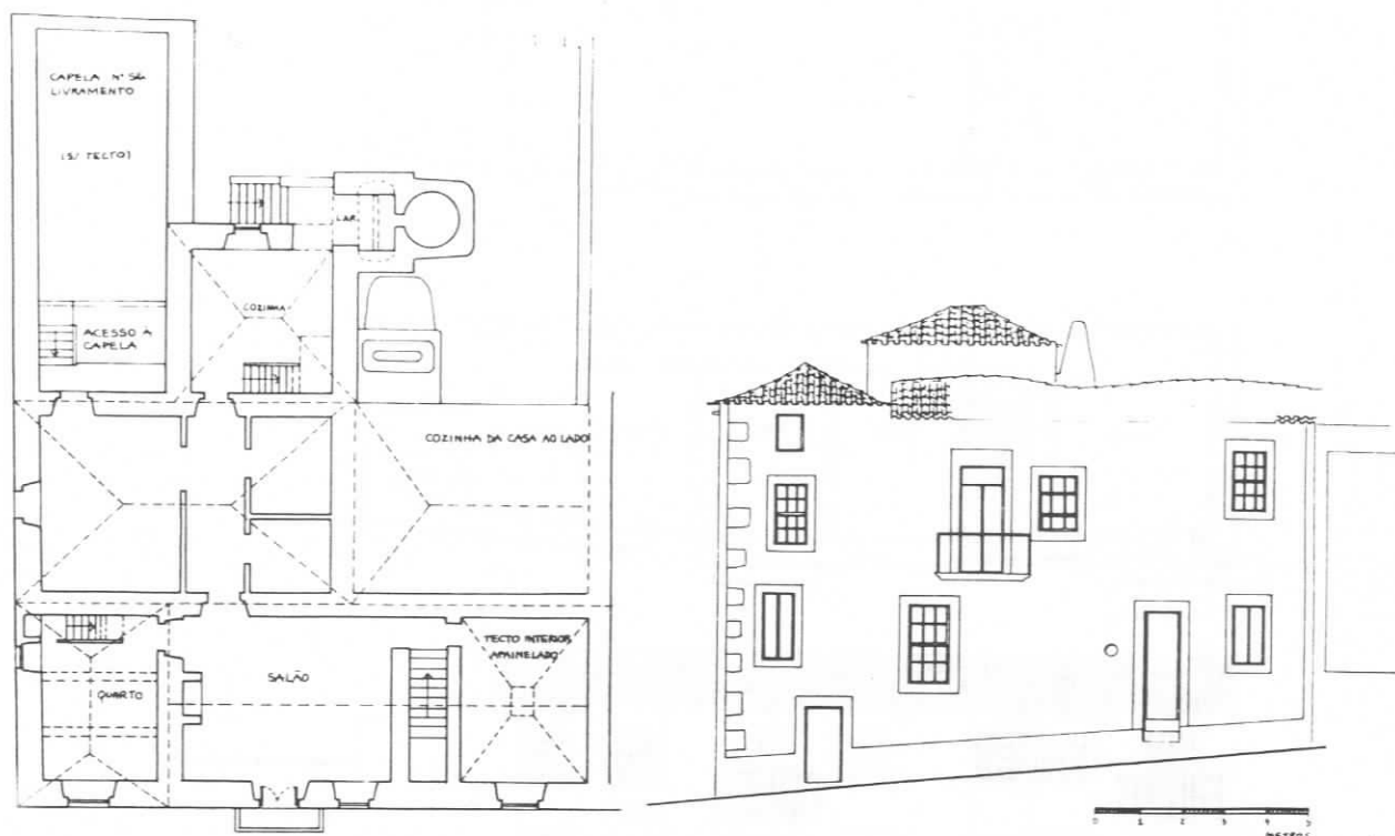
FIG.228 - Santa Maria, Vila do Porto. In FERNANDES [et al.] [210] Açores, ficha n.29 Esc. 1/200
