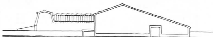
FIG.310 - Graciosa, Caparacho. In FERNANDES [et al.] [210] Açores, ficha n.104. Arquivo. esc. 1/200
