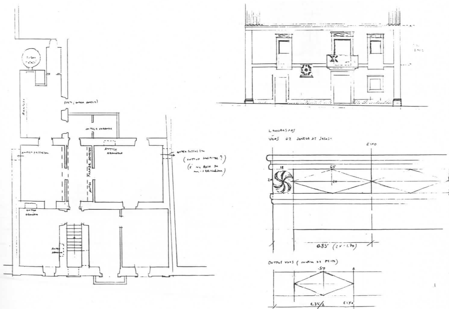
FIG.233 - São Miguel, Ribeira Grande. Levantamento do autor, 1989 Esc. 1/200
