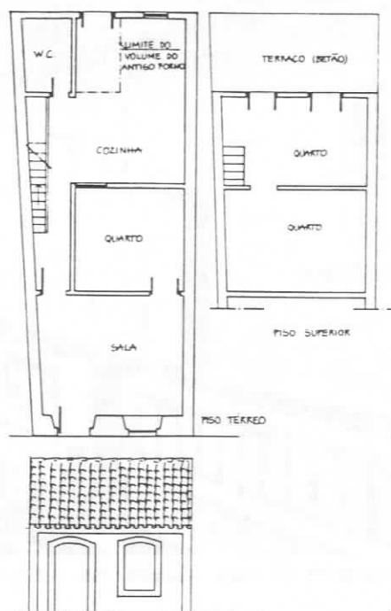
FIG.217 - Angra, casa na rua Nova. In FERNANDES [153] Angra...pág.71 Esc. 1/200
