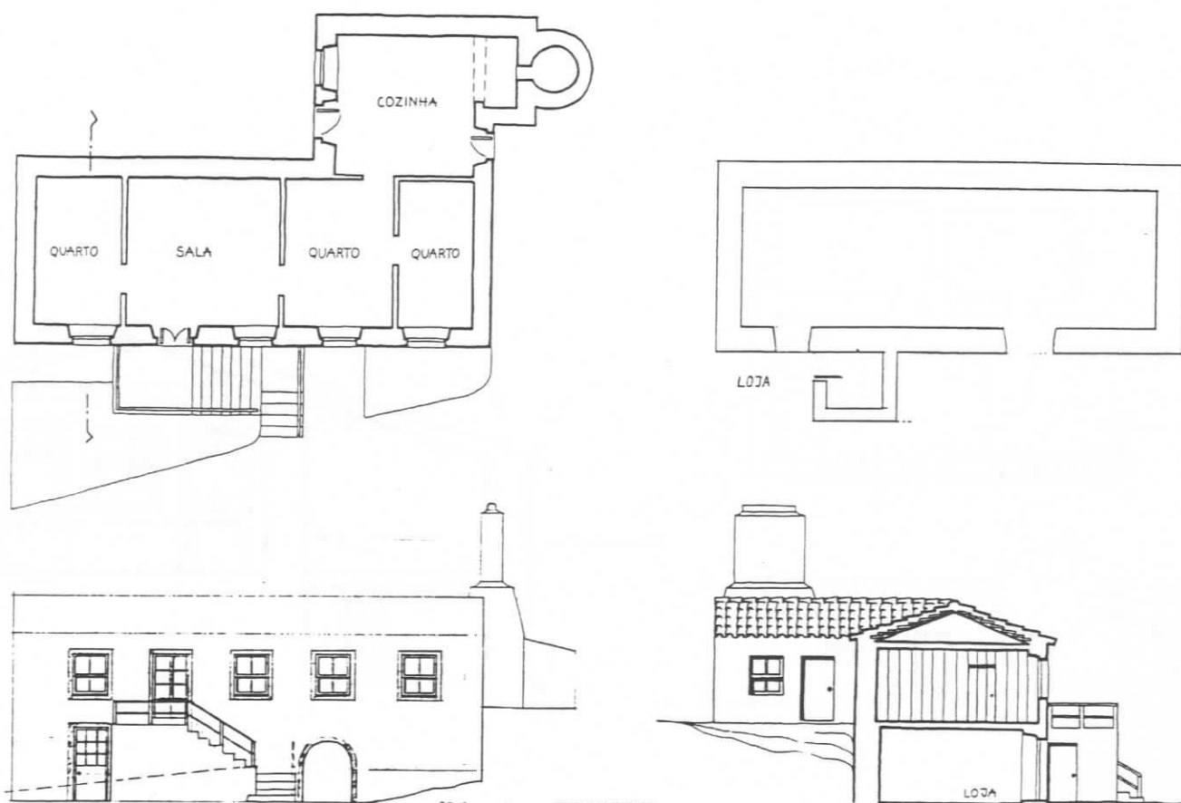
FIG.321 - Flores, Mosteiro. In FERNANDES [et al.] [210] Açores, ficha n.37. Levantamento. Esc. 1/200
