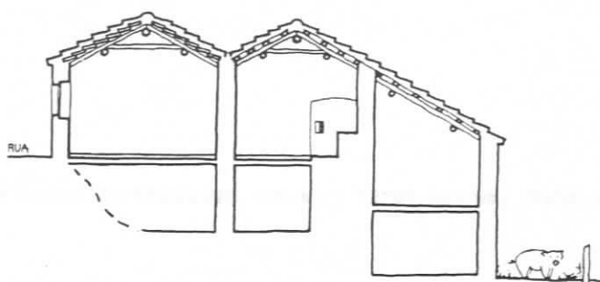
FIG.312 - São Miguel, Agua Retorta. In FERNANDES [et al.] [210] Açores, ficha n.218. Arquivo. Esc. 1/200
