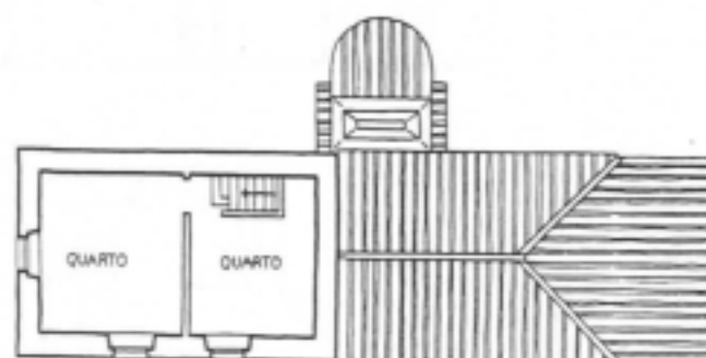
FIG.335 - Santa Maria, Santana. In FERNANDES [et al.] [210] Açores, ficha n.46A. Levantamento. Esc. 1/200
