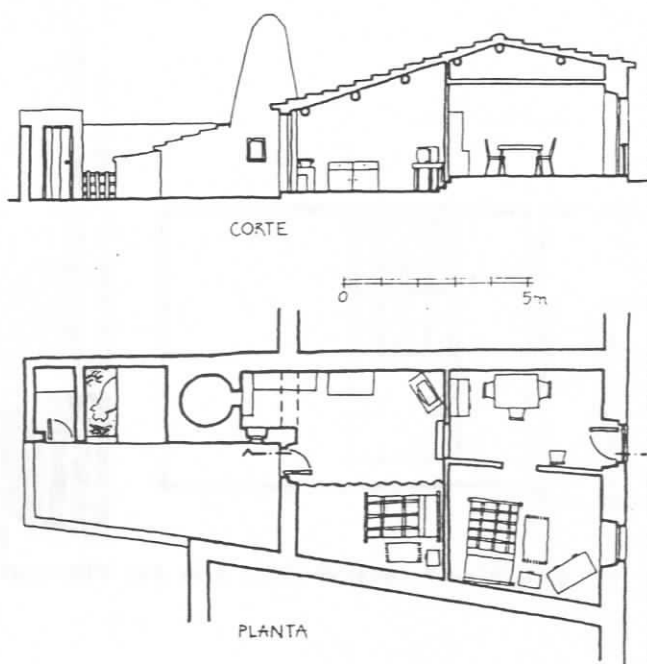
FIG.218 - São Miguel, casa na Ribeira Seca In FERNANDES [et al.] [210] Açores ficha n.172, Arquivo. Esc.1/200
