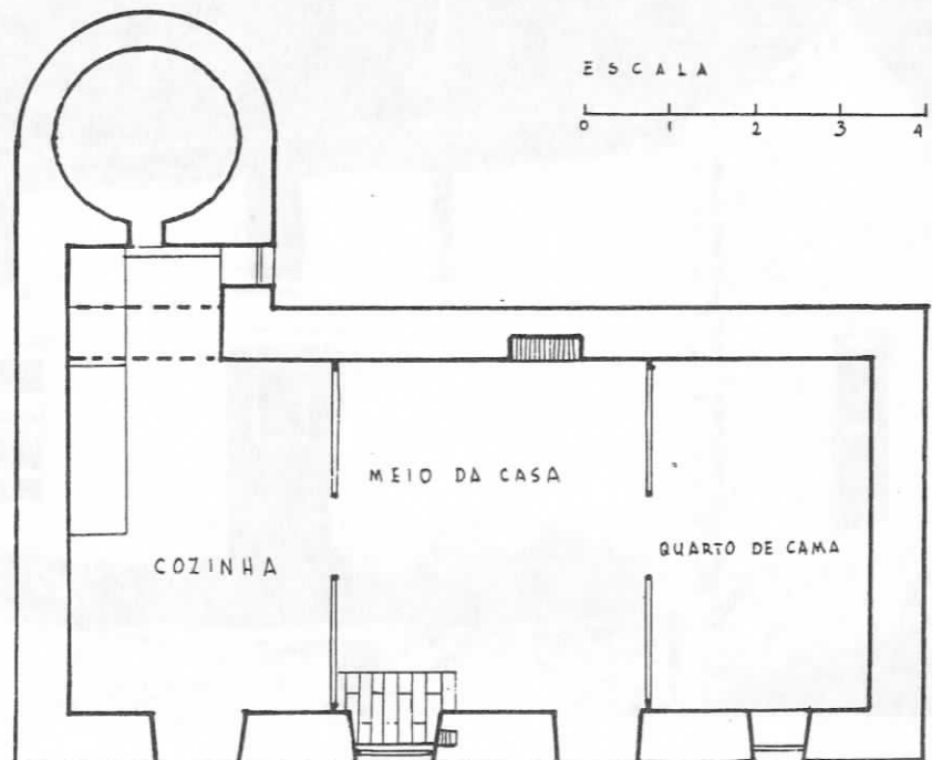
FIG.260 - Ilha Terceira: O "meio da casa". In MACEDO [191] Arquitetura...pág.68. Esc.1/100
