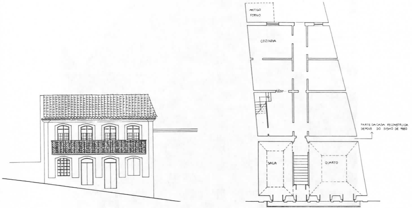
FIG.238 - Angra, casa na rua do Galo. In FERNANDES [153] Angra...pág.76 Esc. 1/200
