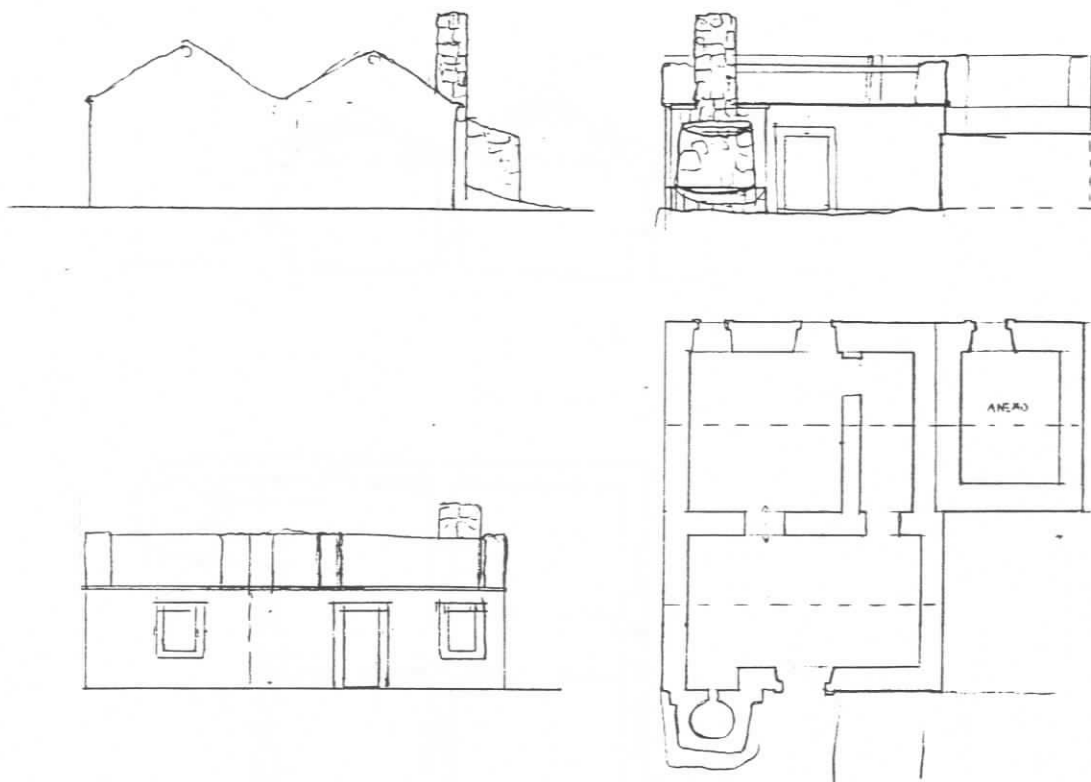
FIG. 345 - Porto Santo, Vila Baleira, "casa do Bispo do Hawai". Levantamento do autor, 1989. Esc. 1/200
