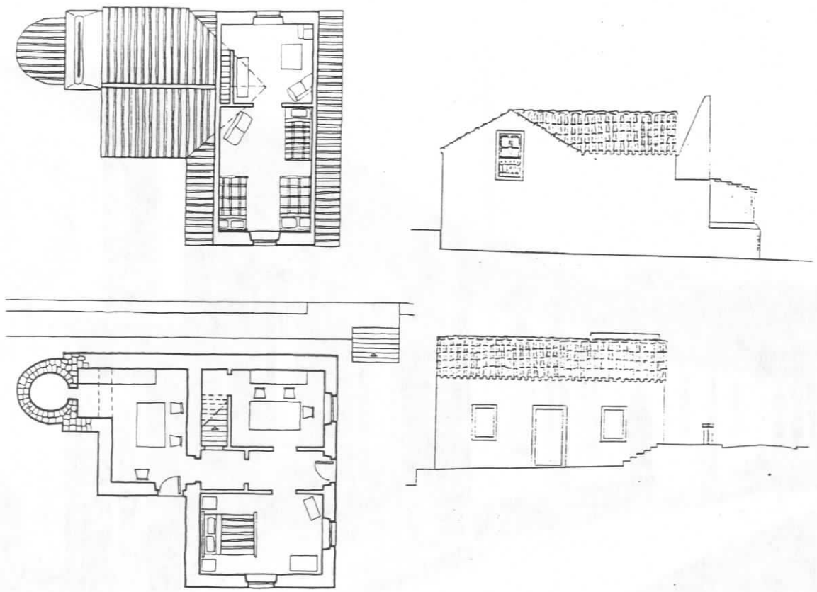
FIG.314 - São Miguel, Feteiras, Canada do Porto. In FERNANDES [et al.] [210] Açores, ficha n.63. Levantamento. Esc. 1/200
