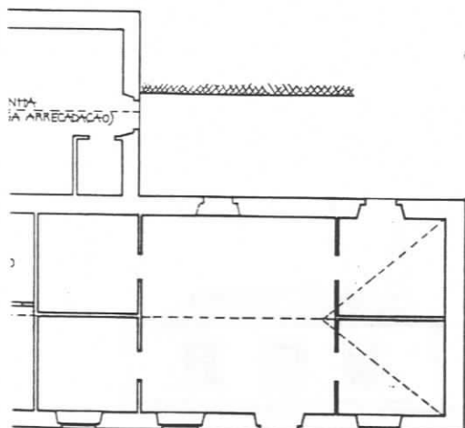
FIG.342 - Terceira, São Sebastião. In FERNANDES [et al.] [210] Açores, ficha n.40, Arquivo. Esc. 1/200
