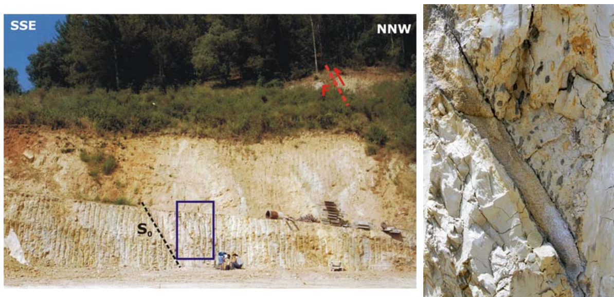
Figura 7 – Corte no Bairro da Mata, a norte de Vila Franca de Xira, em sedimentos miocénicos. A – Aspecto geral, observando-se a estratificação invertida, inclinada para a Falha de Vila Franca de Xira (F). S 0 : N65E, 48NW; B – Pormenor de A, mostrando as tubulações invertidas. Estas tubulações têm cerca de 5 cm de comprimento e 1 cm de diâmetro, estando preenchidas por arenito fino micáceo de cor preta.
