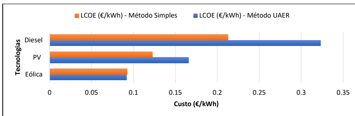
Figura 6.10 - Análise comparativa do LCOE obtido para o caso de estudo utilizando método UAER e método simples
