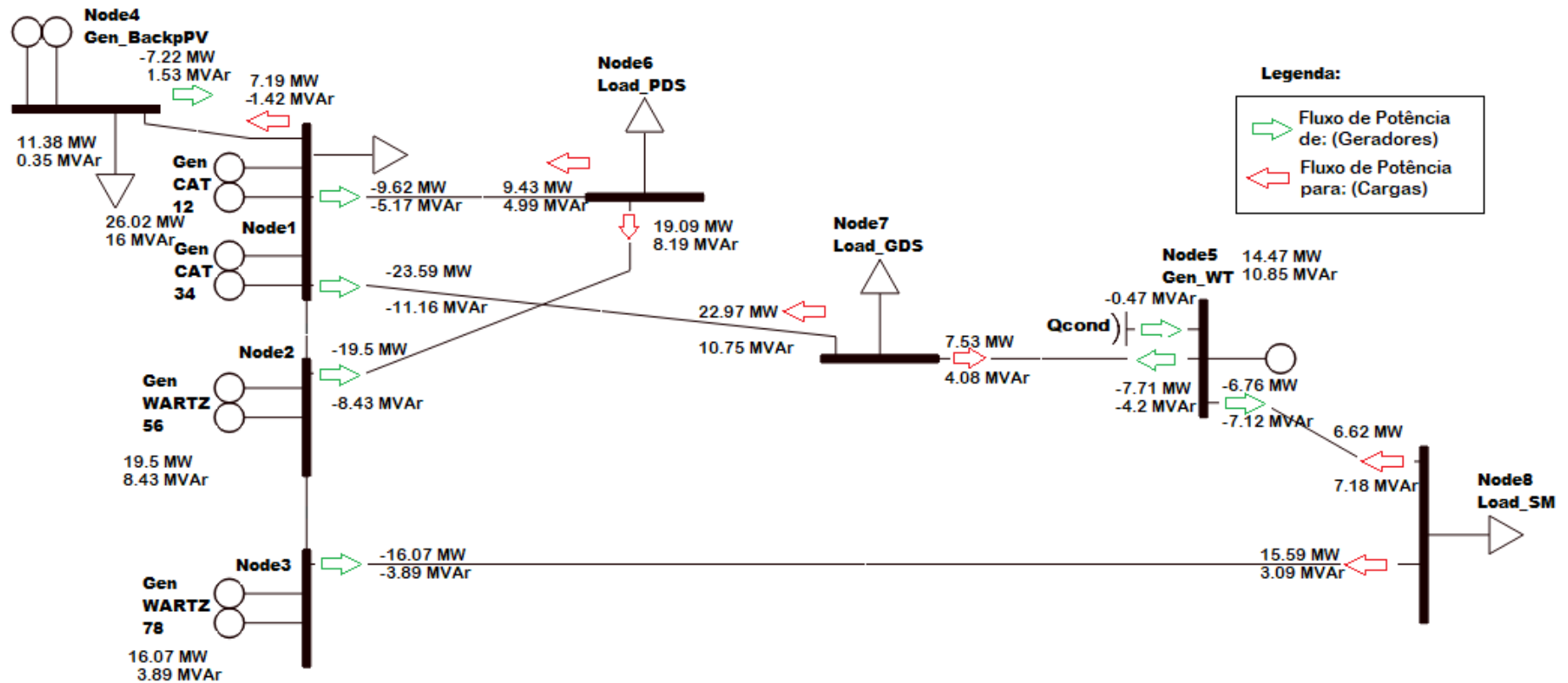
Figura A. 2: Diagrama de potência transitada entre barramentos – Modelo ACOPT – Cenário B (2020)
