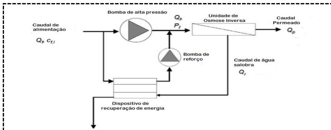
Figura 2.11 - Ilustração da operação de uma unidade de dessalinização RO. Adaptado de [37]
