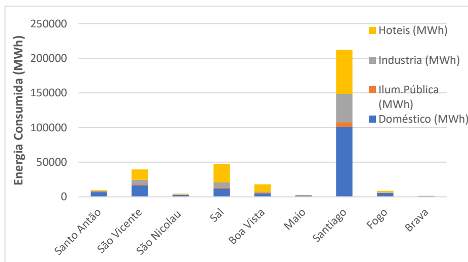
Figura 2.4 - Distribuição do consumo sectorial por ilha. Fonte: [15]
