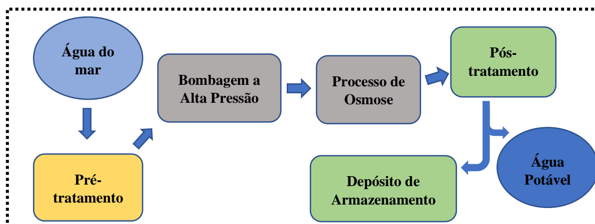
Figura 2.12 - Representação esquemática das etapas inerentes ao processo de dessalinização – RO. Adaptado de [41]
