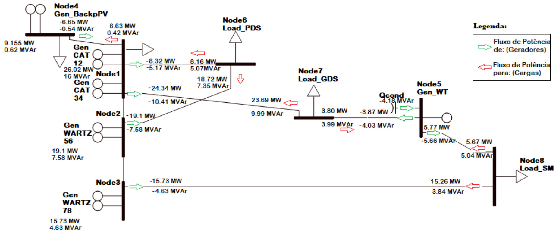
Figura A. 1: Diagrama de potência transitada entre barramentos – Modelo ACOPF – Cenário A (Base)
