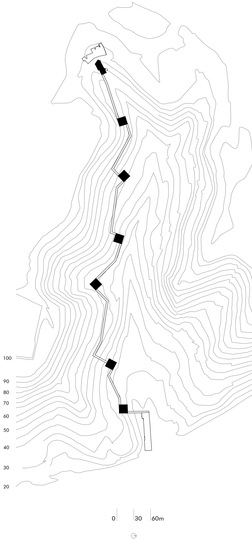
Fig.72 Vale de Torres. Planta. Permanecer
