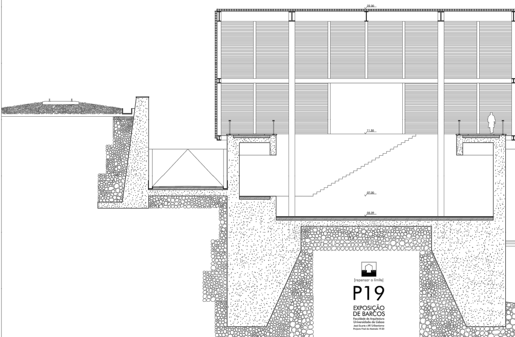
Corte Transversal | Esc. 1:100
