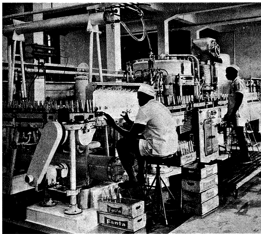
Figura 4. Fábrica de Refrigerantes Mac Mahon, Indústria de Moçambique , vol. 5. n.º 4, 1972, p. 1. A imagem mostra não apenas toda a complexidade das máquinas fabris, mas também a relação dos operários com a dinâmica produtiva. Atentos, equipados num ambiente higienizado onde preponderam as regras de segurança e prevenção, os operários cumprem com perícia as suas funções.
