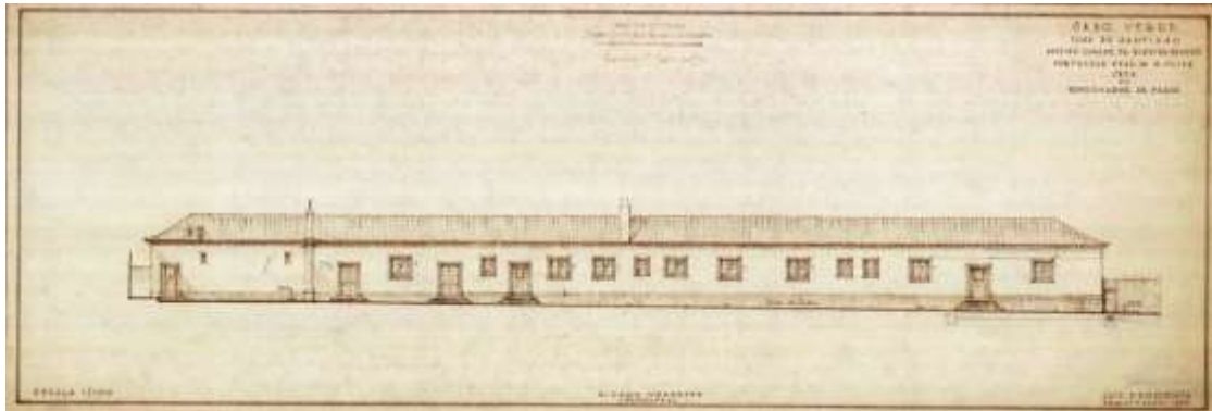
Imagem 56 Projecto não concretizado para a casa do governador da praça, 1969. ANTT, FLB, pt. 2084, doc. 17.
