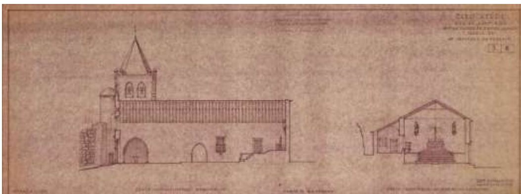
Imagem 77 Corte longitudinal esquerdo e corte transversal no sentido do altar-mor após as obras de restauro projectadas por Luís Benavente, 1969. ANTT, FLB, pt. 2092, doc. 50.
