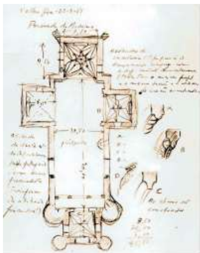
Imagem 263 Levantamento da igreja elaborado pela brigada liderada por Mário Chicó, 1951. FMS, FAMC, pt. 05493.015.004
