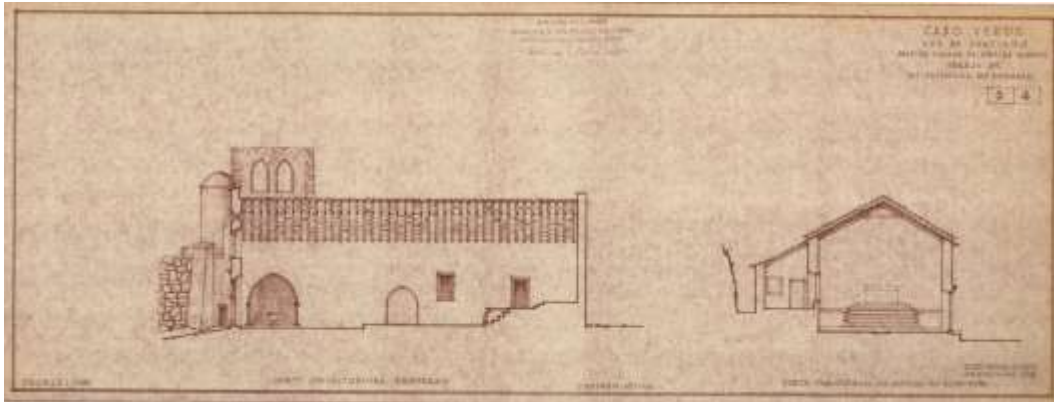
Imagem 76 Levantamento com corte longitudinal esquerdo e corte transversal no sentido do altar-mor antes do restauro, 1969. ANTT, FLB, pt. 2092, doc. 40.
