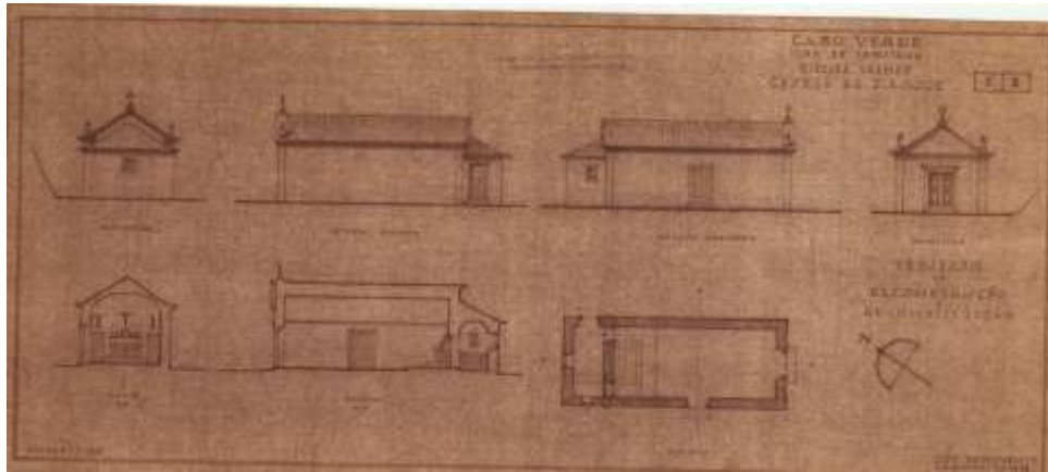
Imagem 52 Projecto de reconstituição da capela de São Roque pelo arquitecto Luís Benavente, 1966. ANTT, FLB, pt. 2081, doc. 12.
