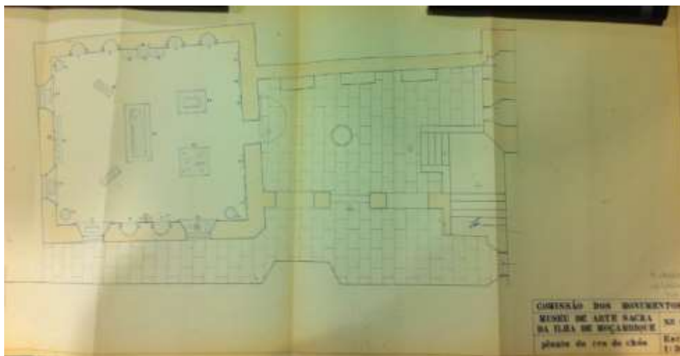
Imagem 207 Planta do rés-do-chão do antigo hospital da Misericórdia/Museu de Arte Sacra, o qual, segundo o plano de Quirino da Fonseca, deveria receber pintura, talha, paramentos e panejamentos. FCG, ASC, Processo 01891.
