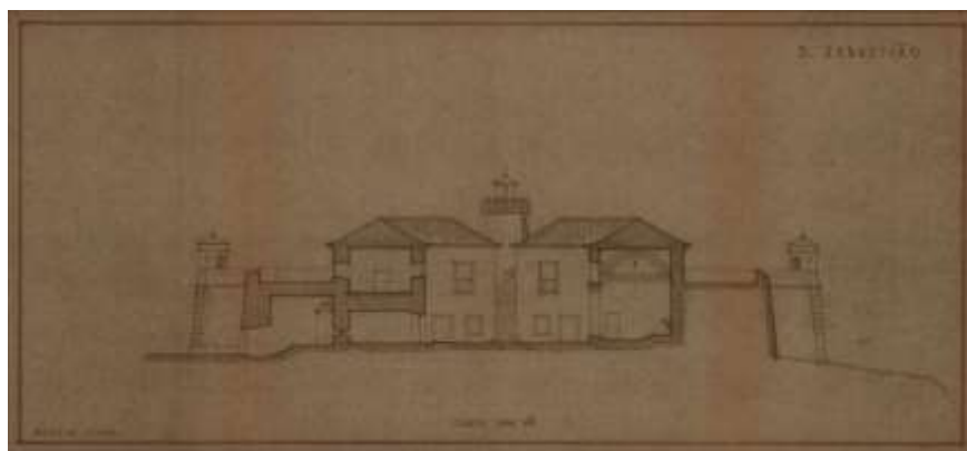
Imagem 23 Corte da fortaleza de São Sebastião, s/d. ANTT, FLB, cx. 70, pt. 490, doc. 1.
