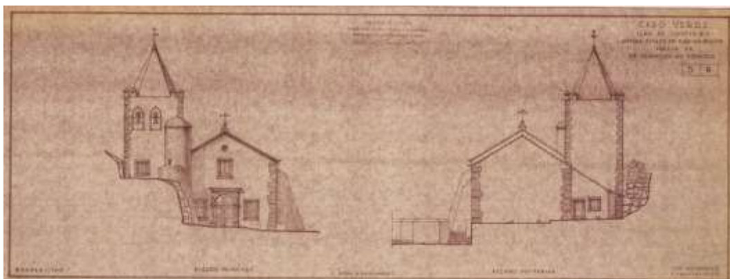
Imagem 75 Projecto de Luís Benavente para o restauro do alçado principal e posterior da igreja de Nossa Senhora do Rosário, 1969. ANTT, FLB, pt. 2092, doc. 44.
