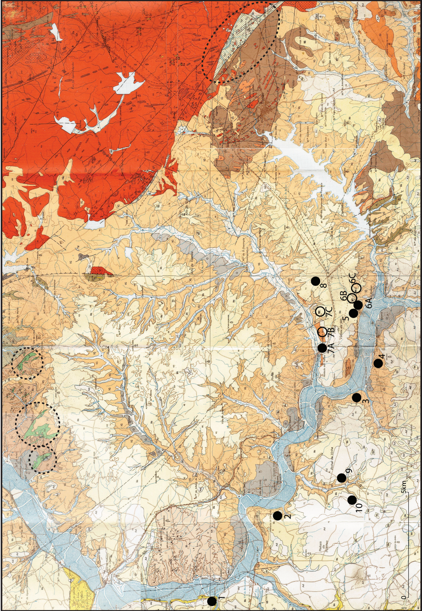
Fig. 2D - Extracto da Carta Geológica de Portugal. Folha 39-D Torreão. Levantada por Gonçalves e Antunes, 1992, na esc. 1:50.000.
