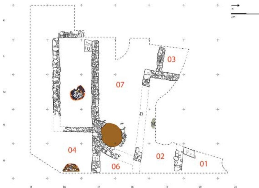
Fig 4. Proposta da 2ª fase de construção do conjunto arquitectónico pré-romano da Rua dos Correios.
