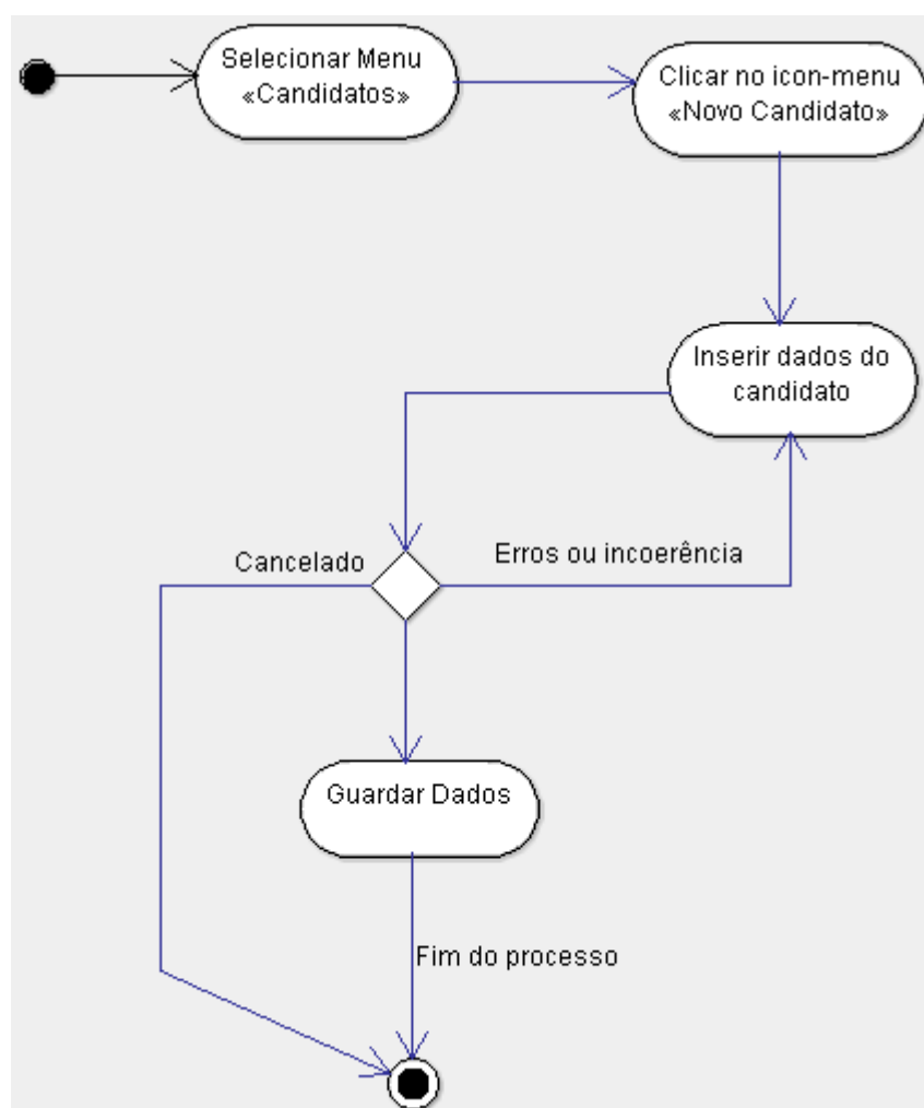
Figura 3-Diagrama de atividade «Novo candidato»
