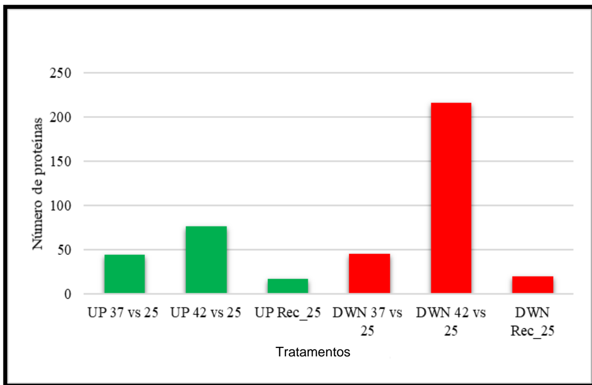
Figura 13- Análise comparativa referente ao número de proteínas menos e mais abundantemente expressas face ao controlo, em Coffea arabica cv Itacu.
