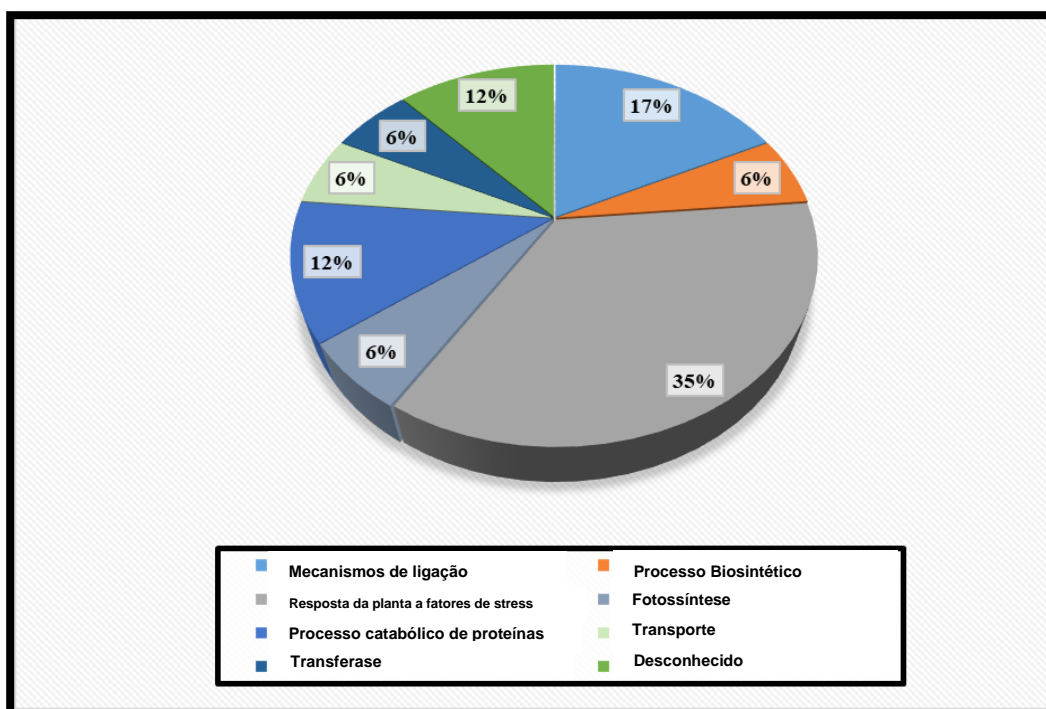
Figura 23- Categorização ontológica das proteínas mais abundantes em Coffea arabica cv. Itacu no período de recuperação em comparação com o controle a 25°C.
