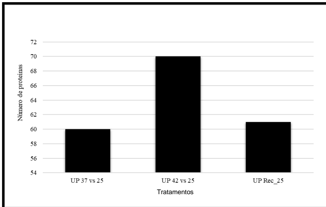
Figura 8- Análise comparativa do número de proteínas mais abundantes com o aumento de temperatura face à temperatura controlo em Coffea canephora cv.CL153. .
