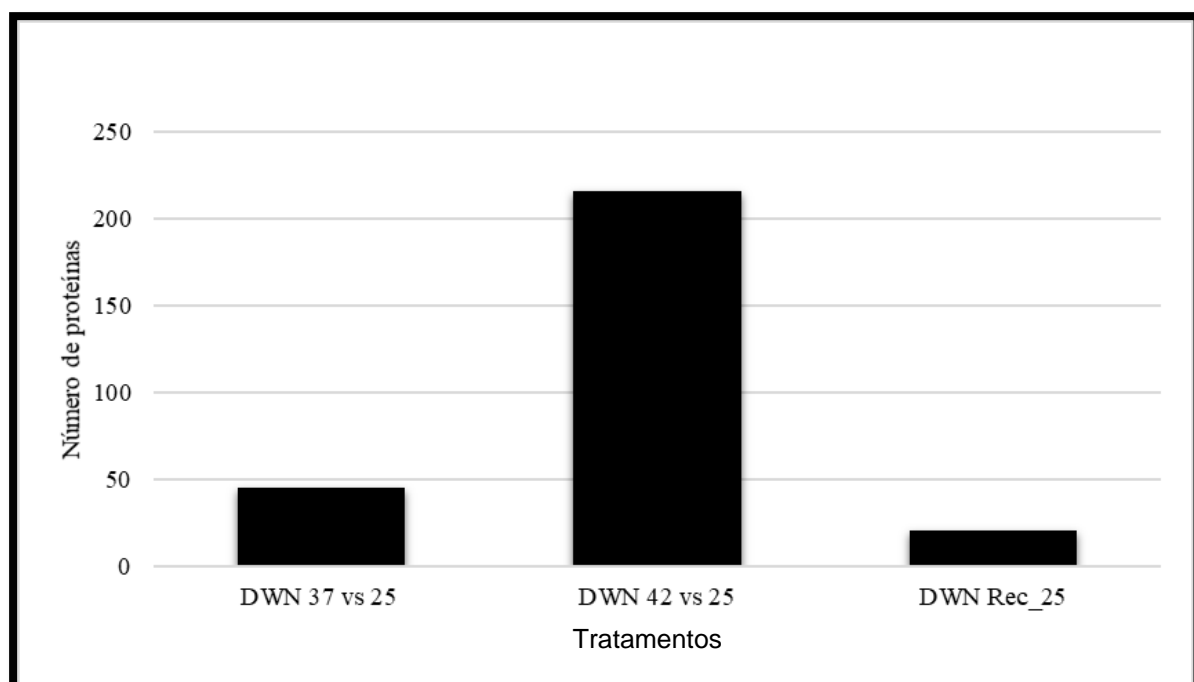
Figura 12- Análise comparativa do número de proteínas menos abundantes com o aumento de temperatura face à temperatura controlo em Coffea arabica cv. Itacu.
