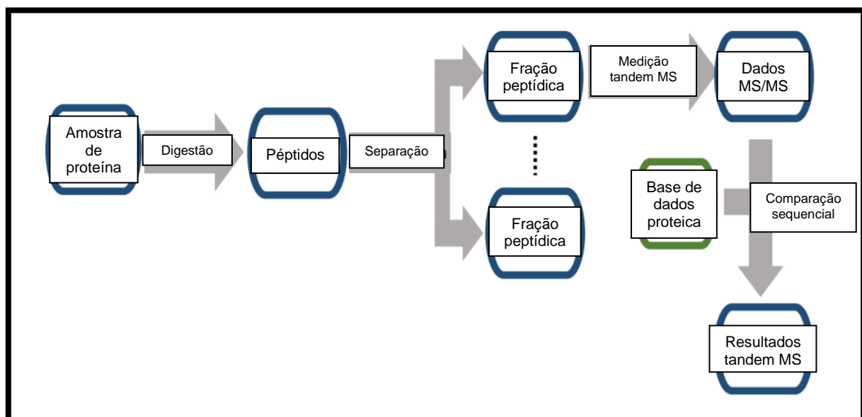
Figura 3- Etapas de identificação de proteínas através do processo de espectrometria tandem (Adaptado de Sequeira et al., 2017).
