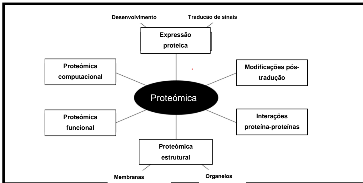
Figura 2 - Tipos e aplicações de estudos em proteômica em diferentes sistemas biológicos. (Adaptado de Vinocur & Altman, 2005).
