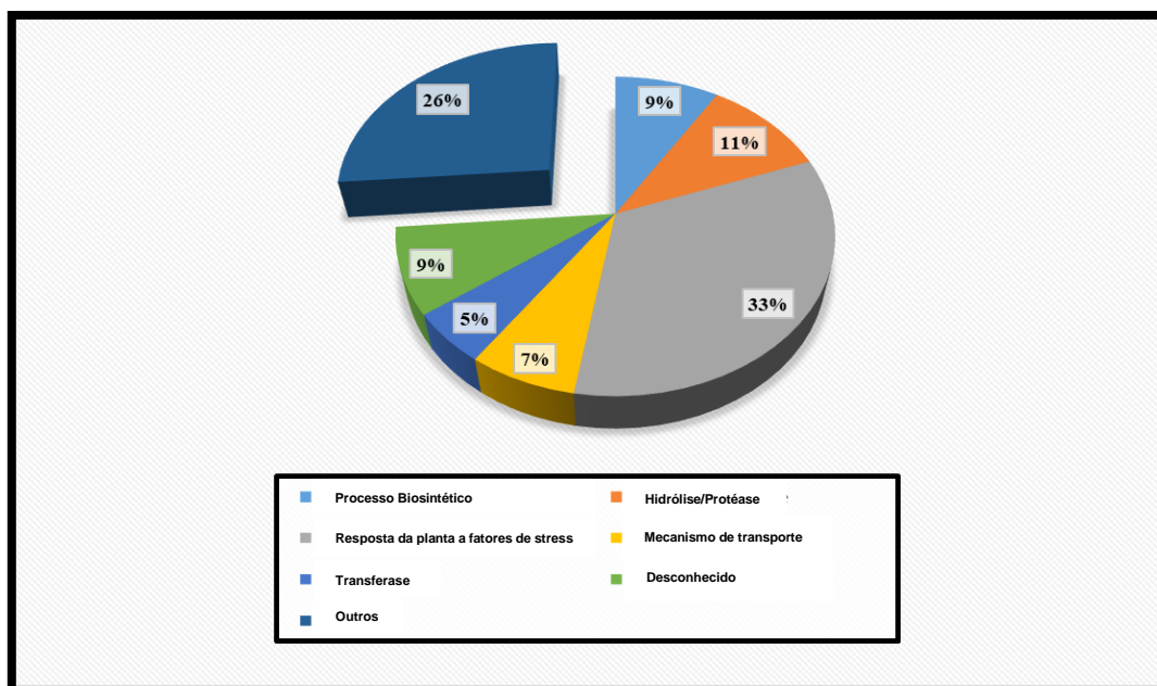
Figura 18- Categorização ontológica das proteínas menos abundantes em Coffea canephora cv. CL153 a 37°C em comparação com o controlo a 25°C.
