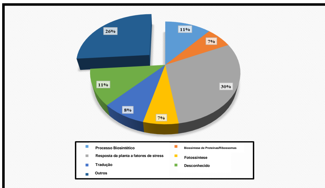
Figura 17- Categorização ontológica das proteínas mais abundantes em Coffea canephora cv. CL153 no período de recuperação em comparação com o controlo a 25°C.
