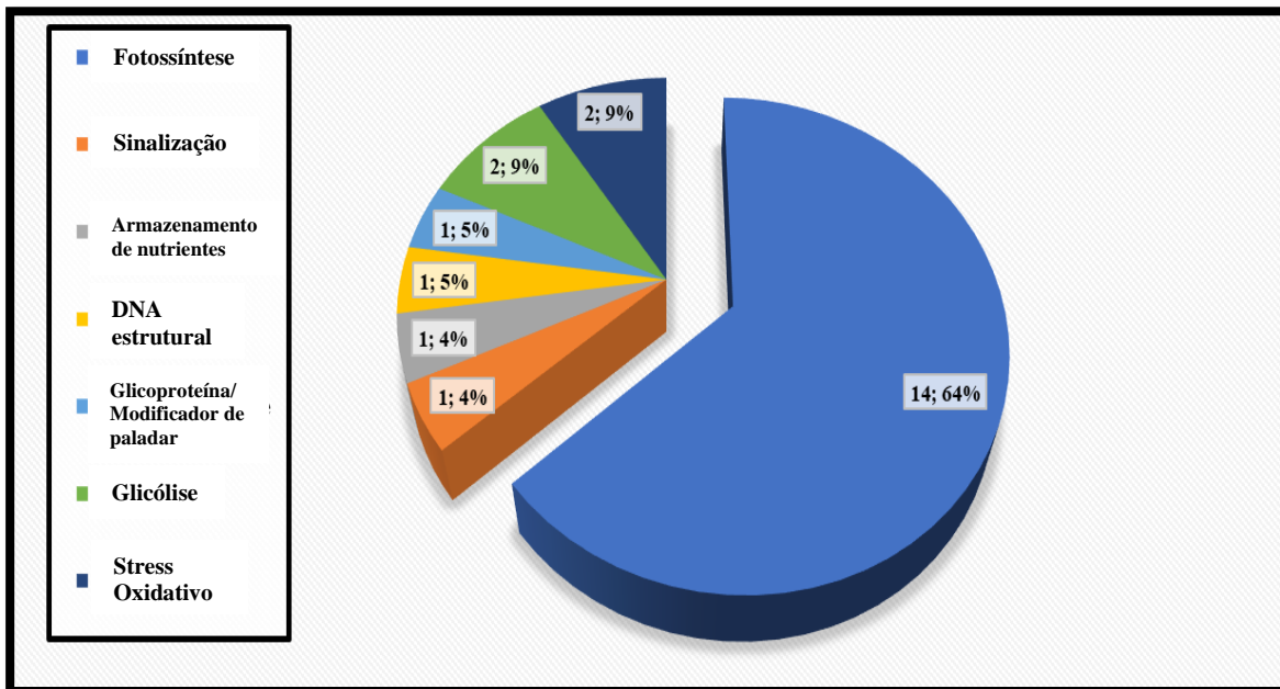
Figura 7- Categorização ontológica das proteínas mais representativas dos dois genótipos.
