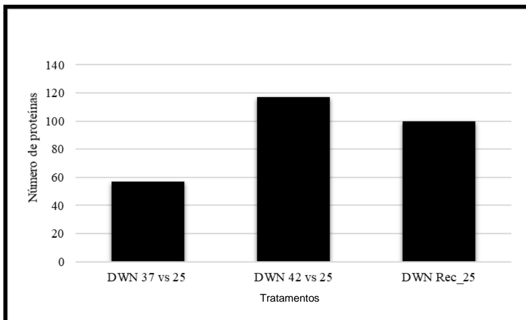
Figura 9- Análise comparativa do número de proteínas menos abundantes com o aumento de temperatura face à temperatura controlo em Coffea canephora cv.CL153.
