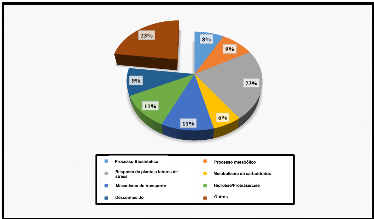
Figura 20- Categorização ontológica das proteínas menos abundantes em Coffea canephora cv. CL153 no período de recuperação em comparação com o controle a 25°C.
