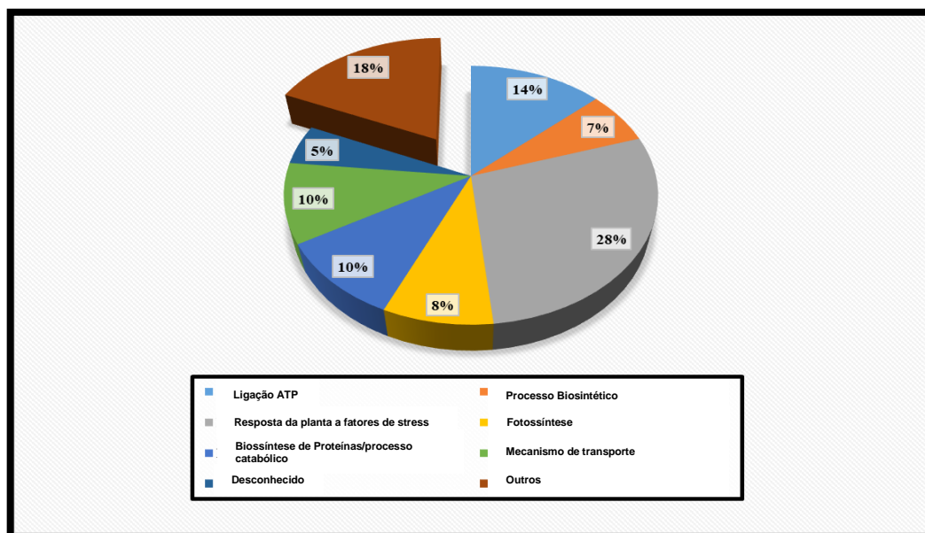
Figura 15- Categorização ontológica das proteínas mais abundantes em Coffea canephora cv. CL153 a 37°C em comparação com o controlo a 25°C.
