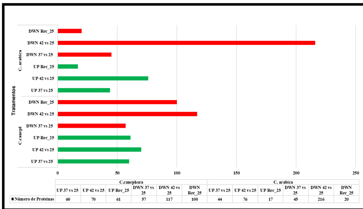
Figura 14- Síntese comparativa da menor e maior abundância de proteínas em Coffea canephora cv. CL153 e Coffea arabica cv. Itacu após os distintos tratamentos térmicos.
