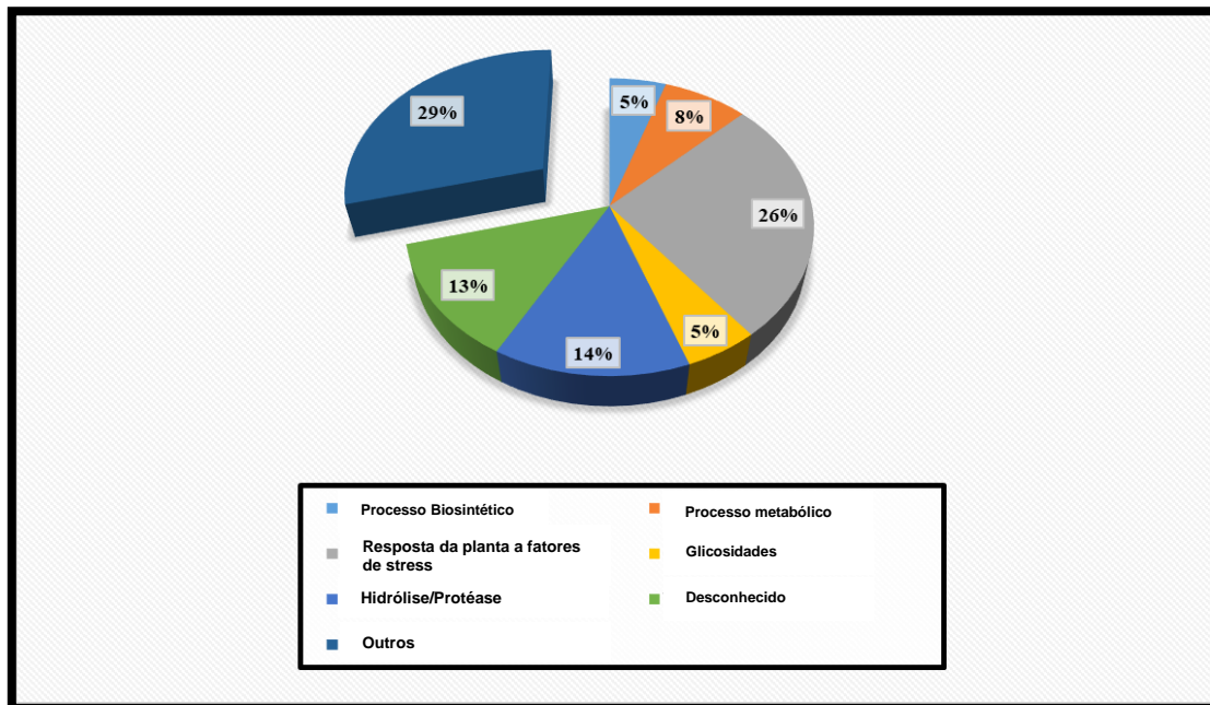
Figura 19- Categorização ontológica das proteínas menos abundantes em Coffea canephora cv. CL153 a 42°C em comparação com o controle a 25°C.
