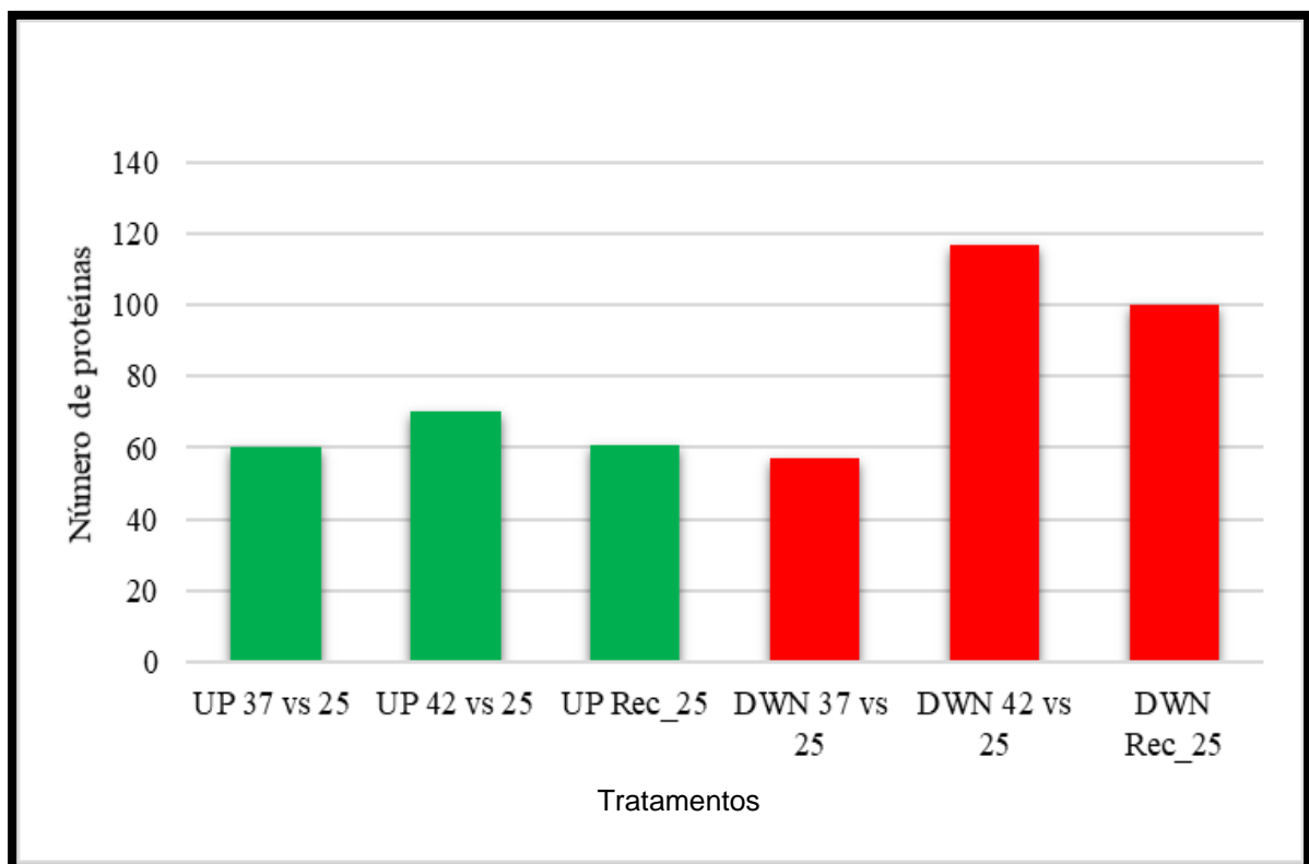
Figura 10- Análise comparativa referente ao número de proteínas menos e mais abundantemente expressas face ao controlo, em Coffea canephora cv.CL153.
