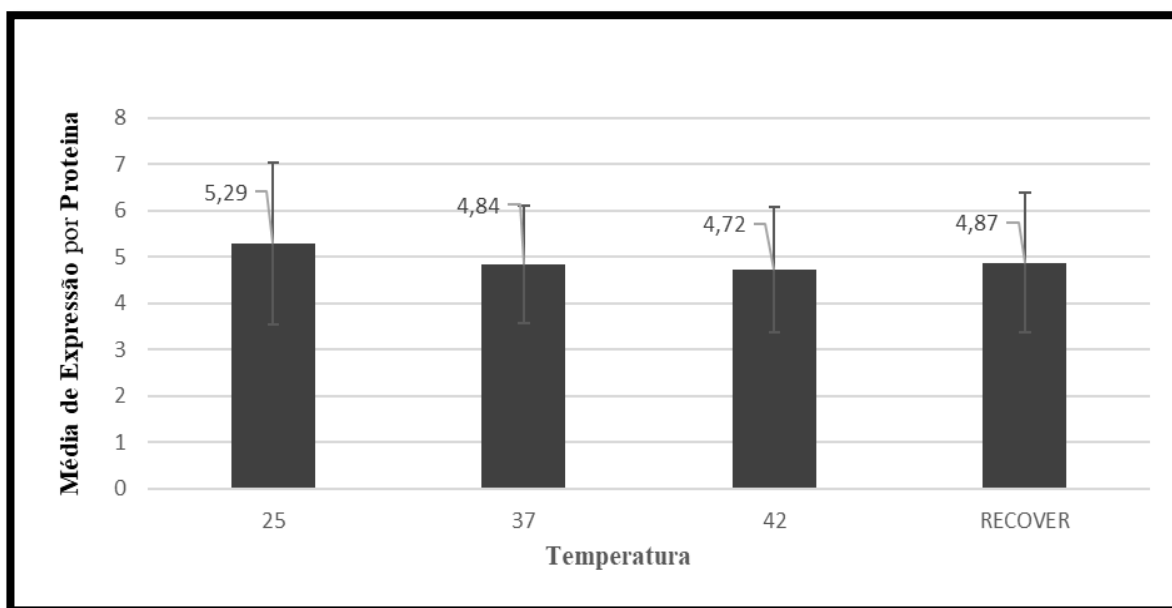
Figura 6- Valores médios da expressão proteica de cada proteína em Coffea arabica (com erro padrão).
