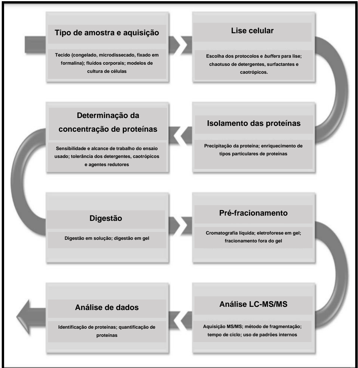
Figura 4- Fluxograma generalizado de uma análise de quantificação proteômica “label free” (Adaptado de Megger et al., 2013).
