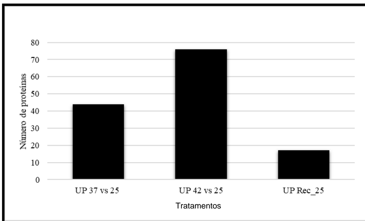
Figura 11- Análise comparativa do número de proteínas mais abundantes com o aumento de temperatura face à temperatura controlo em Coffea arabica cv. Itacu.
