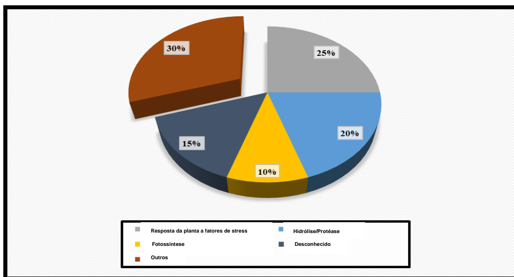
Figura 26- Categorização ontológica das proteínas menos abundantes em Coffea arabica cv. Itacu no período de recuperação em comparação com o controlo a 25°C.
