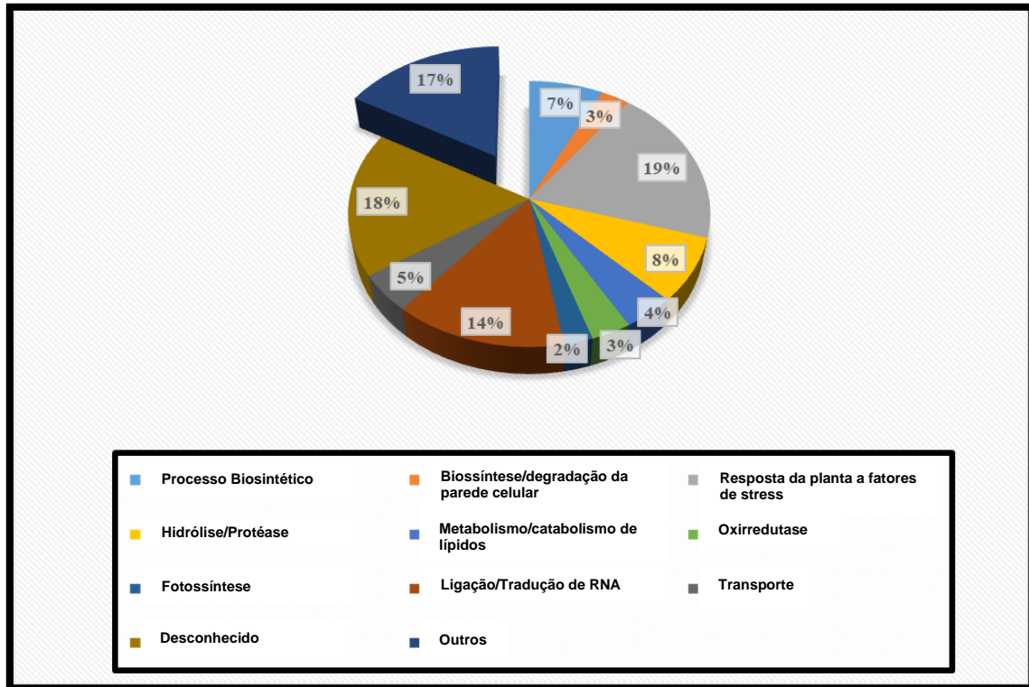
Figura 25- Categorização ontológica das proteínas menos abundantes em Coffea arabica cv.Itacu a 42°C em comparação com o controlo a 25°C.
