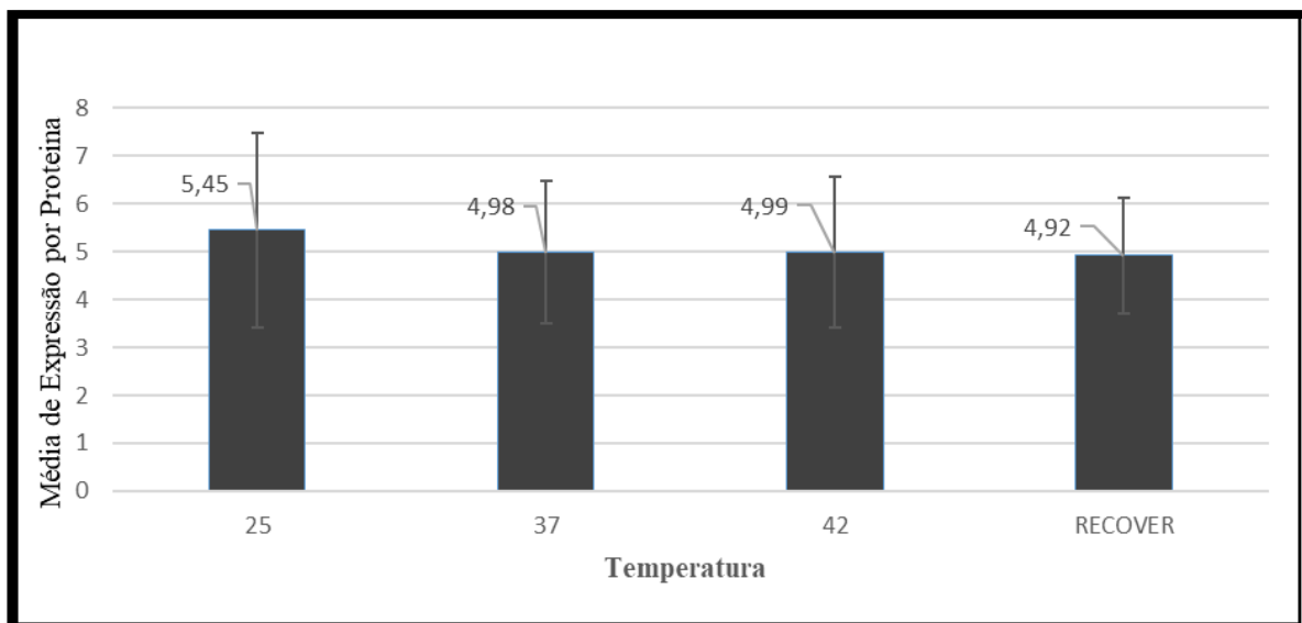
Figura 5- Valores médios da expressão proteica de cada em Coffea canephora (com erro padrão).
