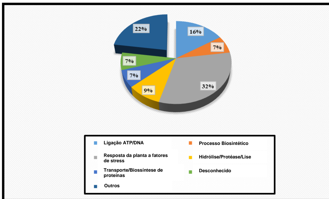
Figura 21- Categorização ontológica das proteínas mais abundantes em Coffea arabica cv. Itacu a 37°C em comparação com o controle a 25°C.
