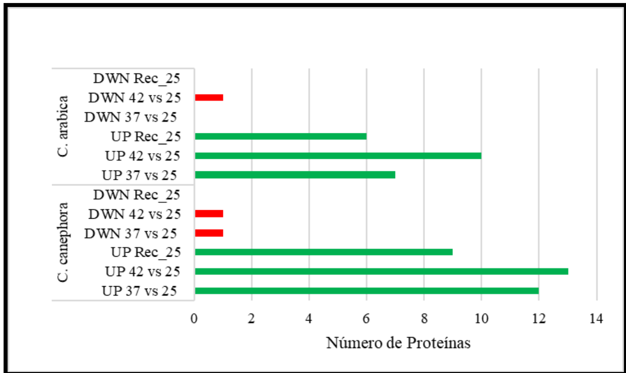
Figura 27- Contabilização de proteínas diretamente relacionadas com respostas da planta ao stress térmico nas variedades Coffea arabica cv. Itacu e Coffea canephora cv. CL153 após os distintos tratamentos de calor.
