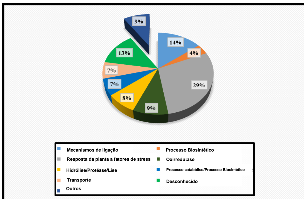
Figura 22- Categorização ontológica das proteínas menos abundantes em Coffea arabica cv. Itacu a 42°C em comparação com o controle a 25°C.
