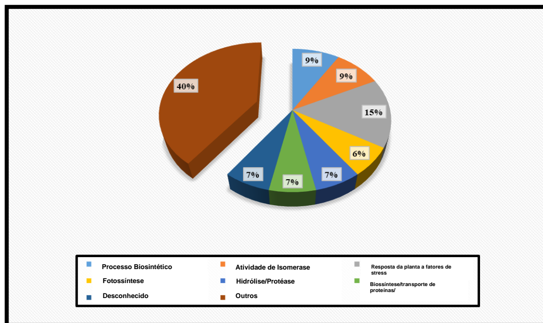
Figura 24- Categorização ontológica das proteínas menos abundantes em Coffea arabica cv. Itacu a 37°C em comparação com o controlo a 25°C.
