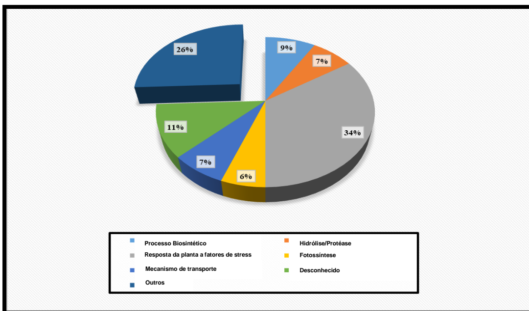
Figura 16- Categorização ontológica das proteínas mais abundantes em Coffea canephora cv. CL153 a 42°C em comparação com o controlo a 25°C.
