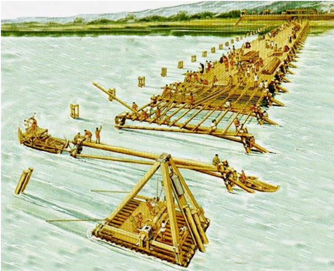
Imagem 14 – Reconstrução do que terá sido a ponte que César mandou construir sobre o rio Reno, em 55 a. C., para entrar em território germano, durante a Guerra das Gálias. Adaptado a partir de: CONNOLLY, Peter. (2016), Greece and Rome at War . Yorkshire: Frontline Books, p. 240.
