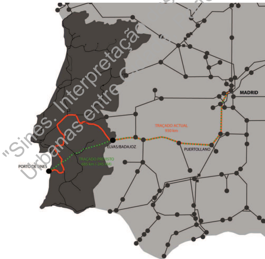
| Imagem 9 | Traçado Ferrovia Mercadorias - Actual e Prevista Detalhe | Fonte. Documentos cedidos pela Administração do Porto de Sines (Adaptado).
