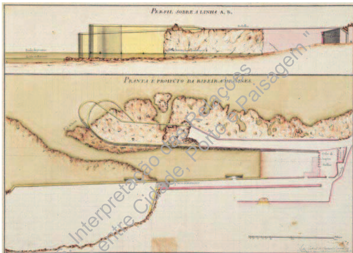
| Cartografia 18 | Planta e Projecto da Ribeira de Sines | 1790 | Autor: CHERMONT, João Gabriel | Fonte: Catálogo Online – Cartoteca do Instituto Geográfico Português, disponível em: http://www.igeo.pt/servicos/cdi/cartoteca/detalheC.asp?cod=103 , consultado a 03 de Março de 2010.
