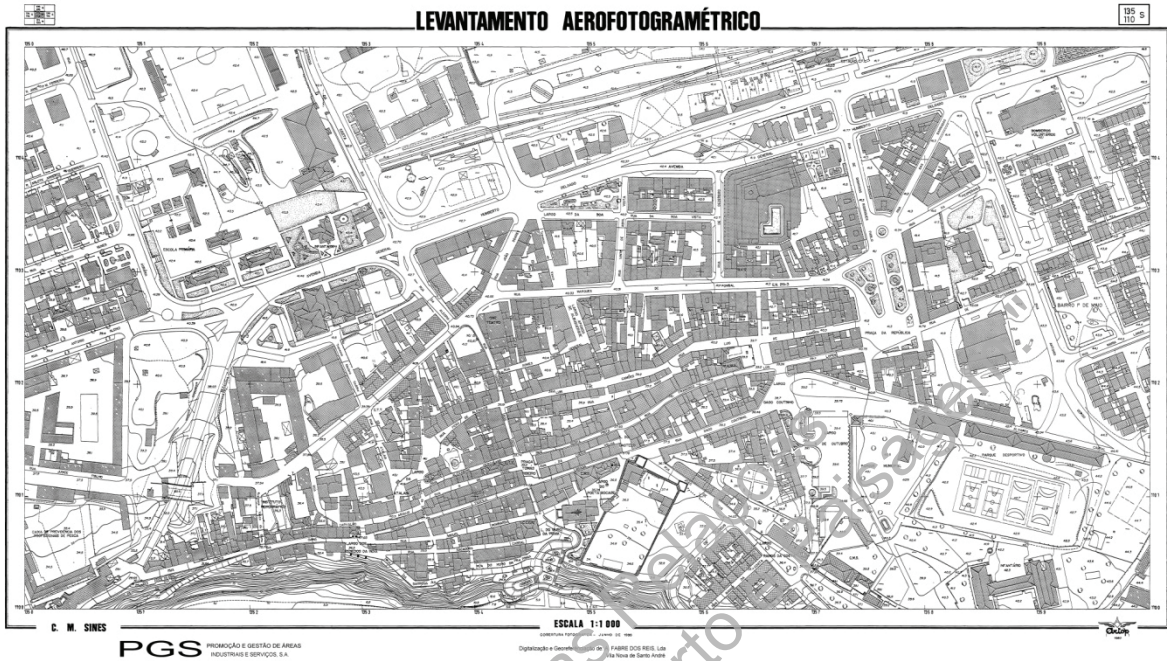
| Cartografia 68 | Sines - Levantamento Aerofotogramétrico | 1983 | Câmara Municipal de Sines e Programação e Gestão de Áreas Industriais e Serviços, S.A. (PGS), Escala: 1:1.000, Folha 135/110/S, Documento Cedido pela Aicep Global Parques.
