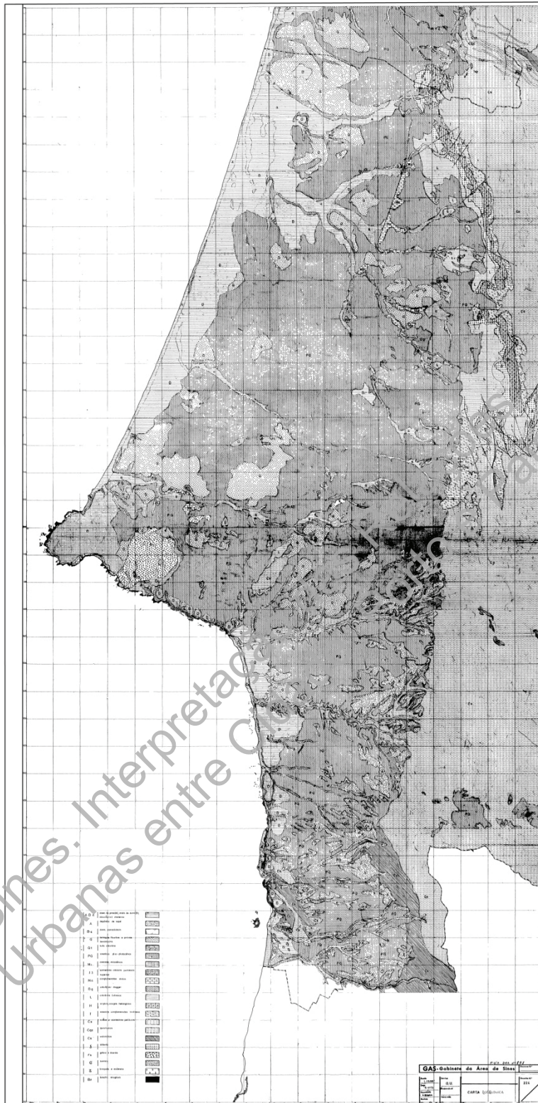
| Cartografia 51 | Carta Geológica | 1972 | Gabinete da Área de Sines, Escala 1:25.000, Documento Cedido pela Aicep Global Parques.
