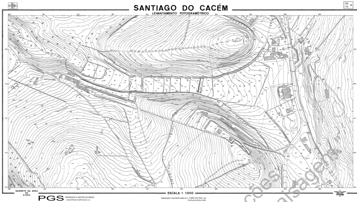
| Cartografia 74 | Santiago do Cacém - Levantamento Aerofotogramétrico | Sem Data | Gabinete da Área de Sines e Programação e Gestão de Áreas Industriais e Serviços, S.A. (PGS), Escala: 1:1.000, Folha 150/115/N, Documento Cedido pela Aicep Global Parques.
