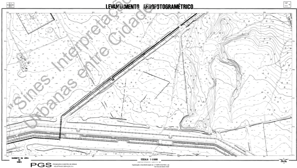
| Cartografia 73 | Sines - Levantamento Aerofotogramétrico | 1982 | Gabinete da Área de Sines e Programação e Gestão de Áreas Industriais e Serviços, S.A. (PGS), Escala: 1:2.000, Folha 137/111/N, Documento Cedido pela Aicep Global Parques.
