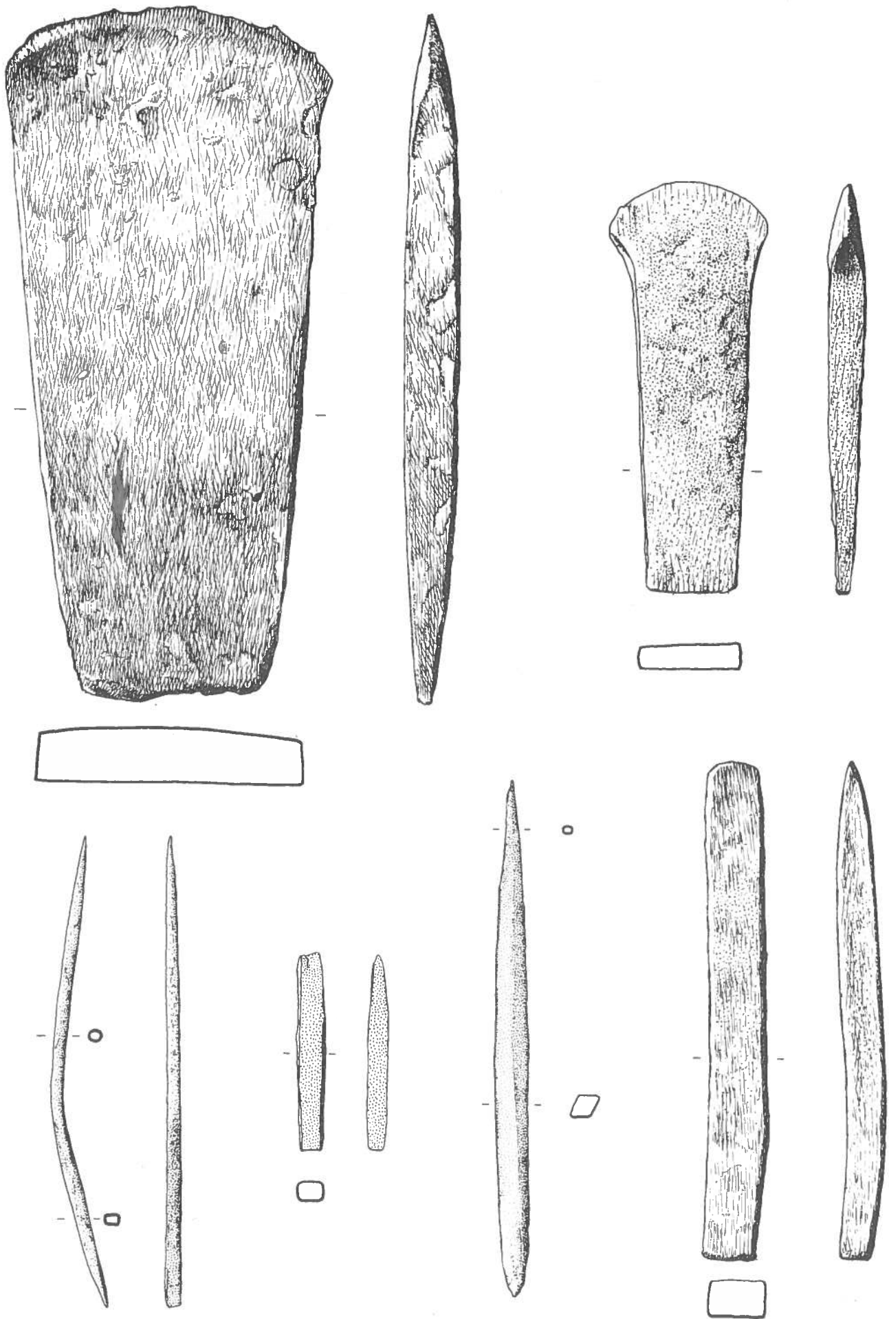
Est. 99. Cerro do Castelo de Santa Justa. Metalurgia (5). 1: machado K.16.-15; 2: machado H.28.-12; 3: furador H.25.-9; 4: escopro M.30.-2; 5: furador G.IJ.-s/n; 6: escopro L.11.-104. 1:1
