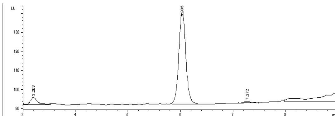
Cromatograma de uma amostra analisada. Simulador água desionizada em contacto com o biberão por 30 minutos a 100°C. TR = 6,035 minutos
