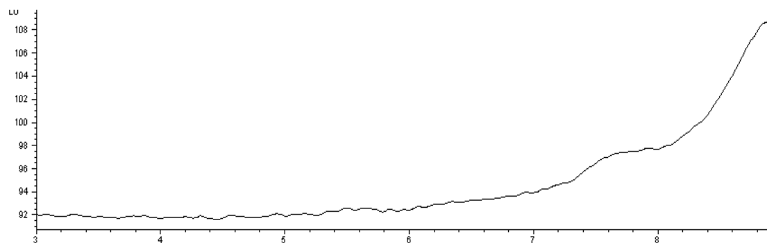
Cromatograma de um branco
