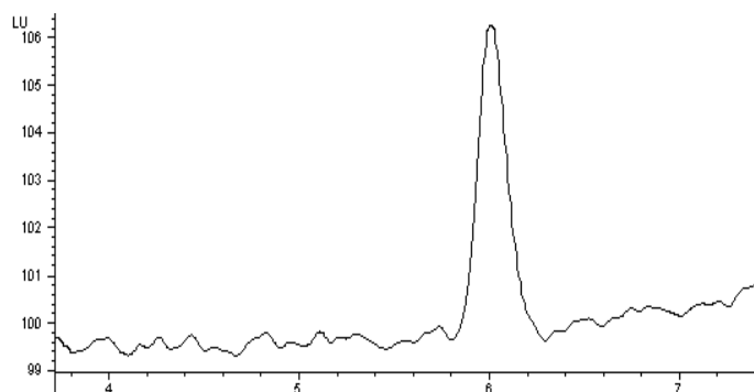
Cromatograma de um padrão de bisfenol A com concentração de 10 ppb; TR = 6,095
