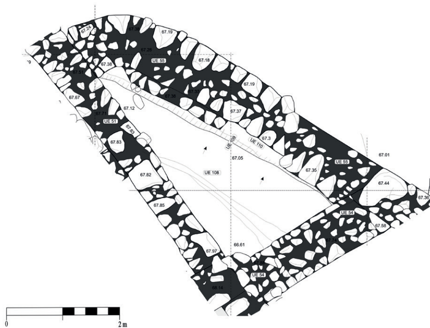
I.148 – Planta do Ambiente 8 da Sondagem 4.
