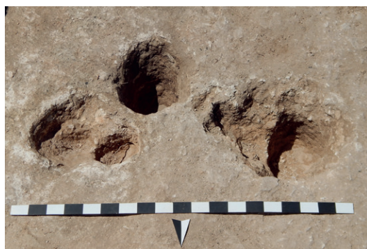
I.51 – Buracos de poste no final da escavação, Ambiente 10.
