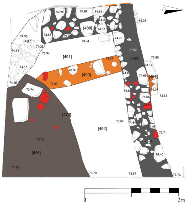
I.100 – Planta do Ambiente 52, Sondagem 8.
