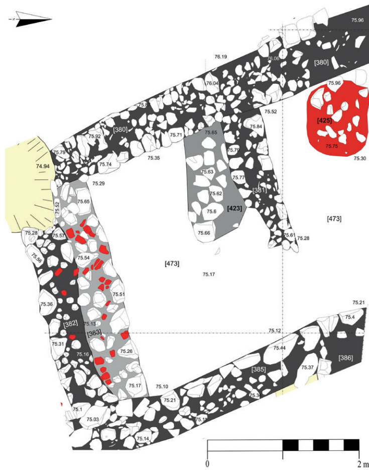
I.86 – Planta final do Ambiente 38, Sondagem 8.
