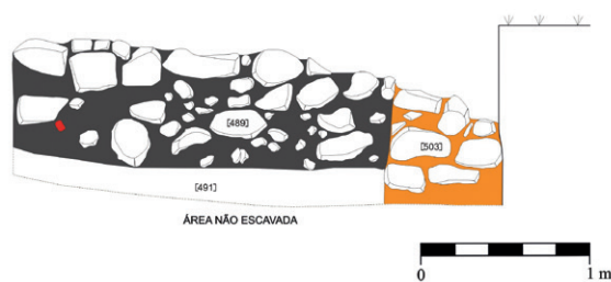
I.98 – Alçado UE [489], Ambiente 52, Sondagem 8.
