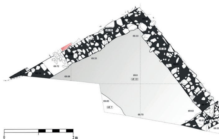
I.141 – Planta do Ambiente 1 da Sondagem 4.
