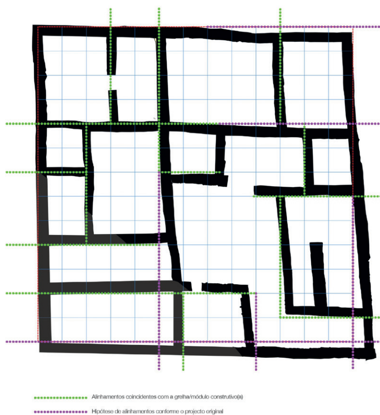
I.171 –Análise do projecto. A verde alinhamentos coincidentes com a grelha/módulo construtivo, a roxo hipótese de alinhamentos conforme o projecto original.
