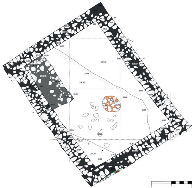
I.161 – Planta do Ambiente 24 da Sondagem 4.
