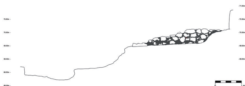
I.58 – Corte e alçado da área de Sondagem 5, correspondendo aos Ambientes 30 e 31.
